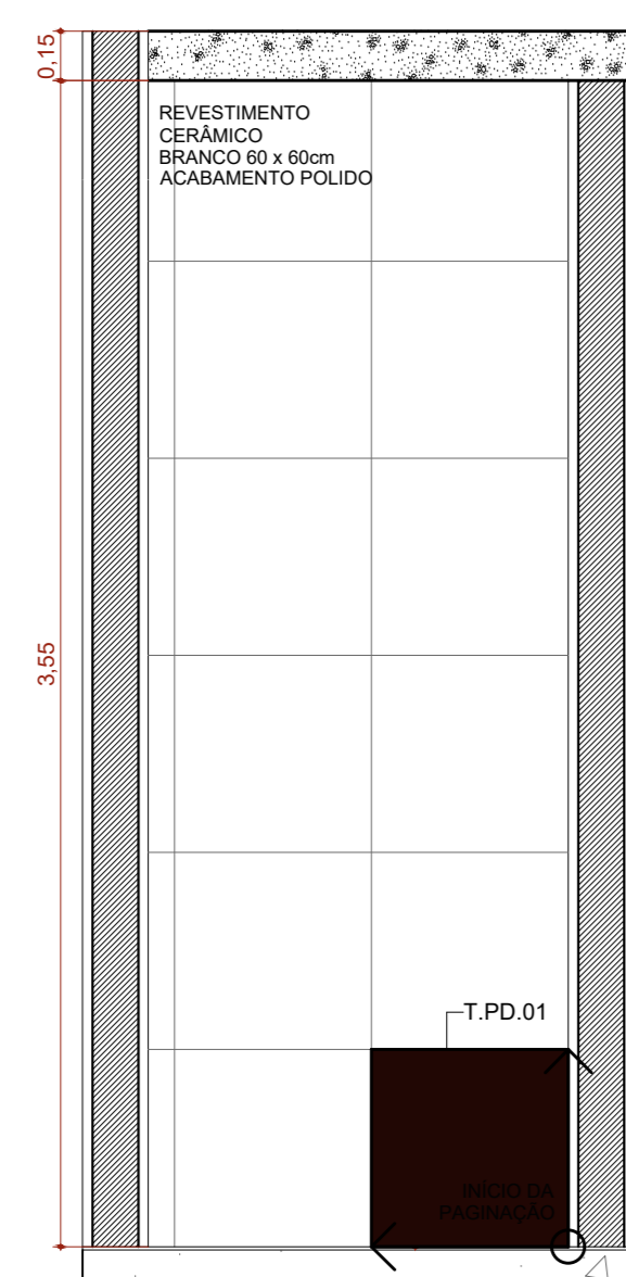
A.M.11 VISTA 01 Escala: 1:25
