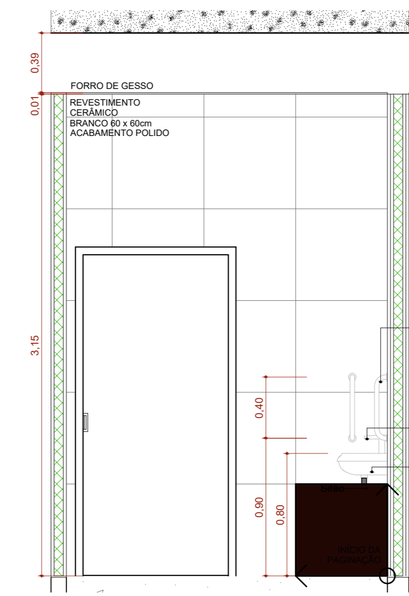
A.M.12 VISTA 03 Escala: 1:25
