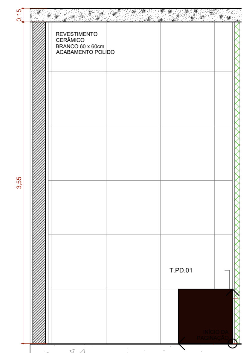
A.M.10 VISTA 02 Escala: 1:25
