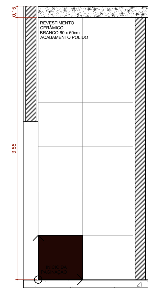
A.M.10 VISTA 01 Escala: 1:25
