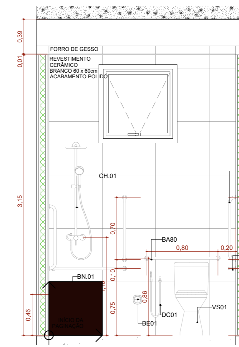
A.M.12 VISTA 04 Escala: 1:25
