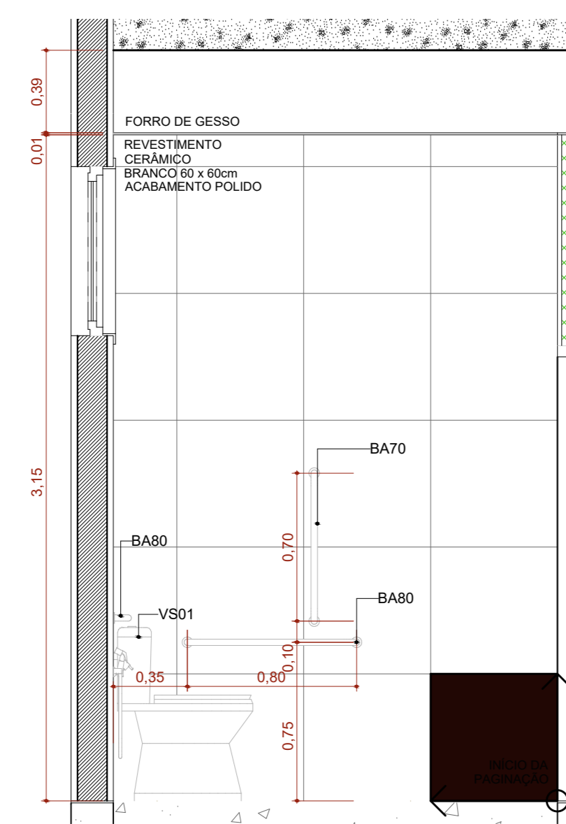
A.M.12 VISTA 01 Escala: 1:25
