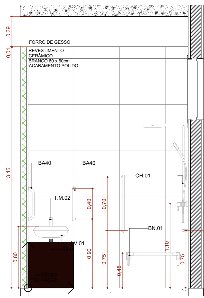
A.M.12 VISTA 02 Escala: 1:25
