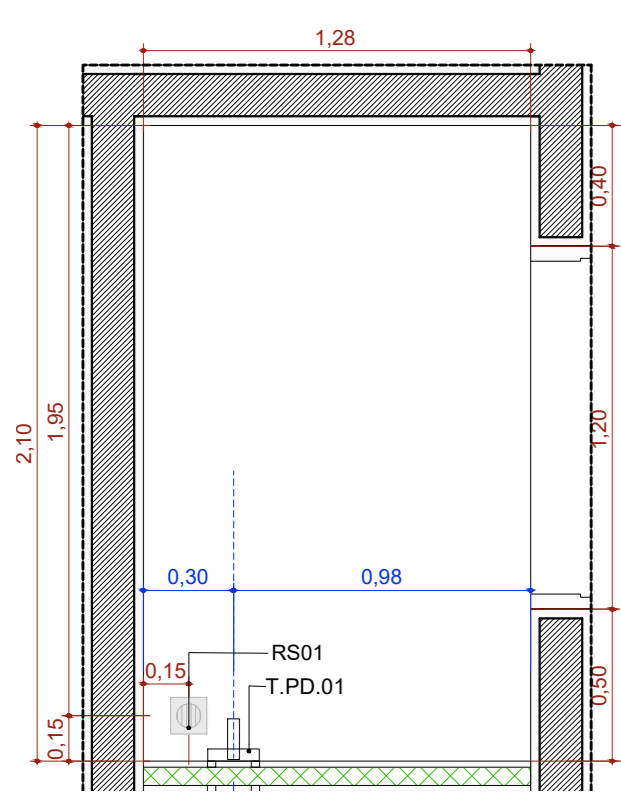
A.M.11 Abrigo de Reíduos comuns (Grupo D) Escala: 1:25
