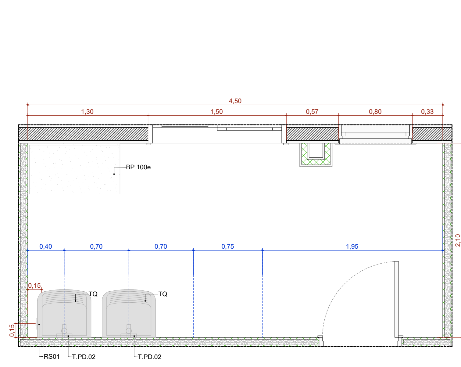
A.M.09 Sala para lavagem de roupas Escala: 1:25
