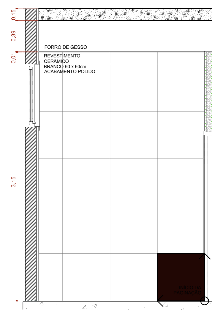
A.M.09 VISTA 01 Escala: 1:25
