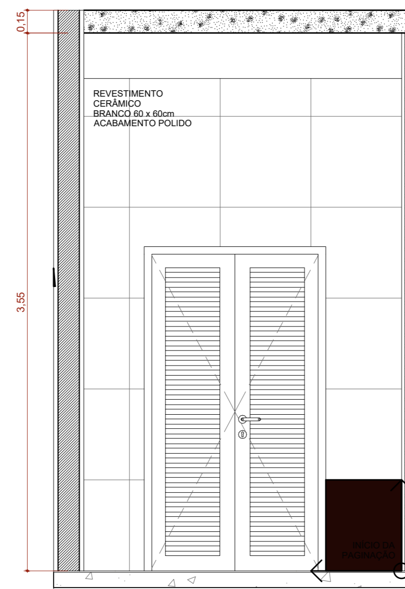
A.M.11 VISTA 02 Escala: 1:25
