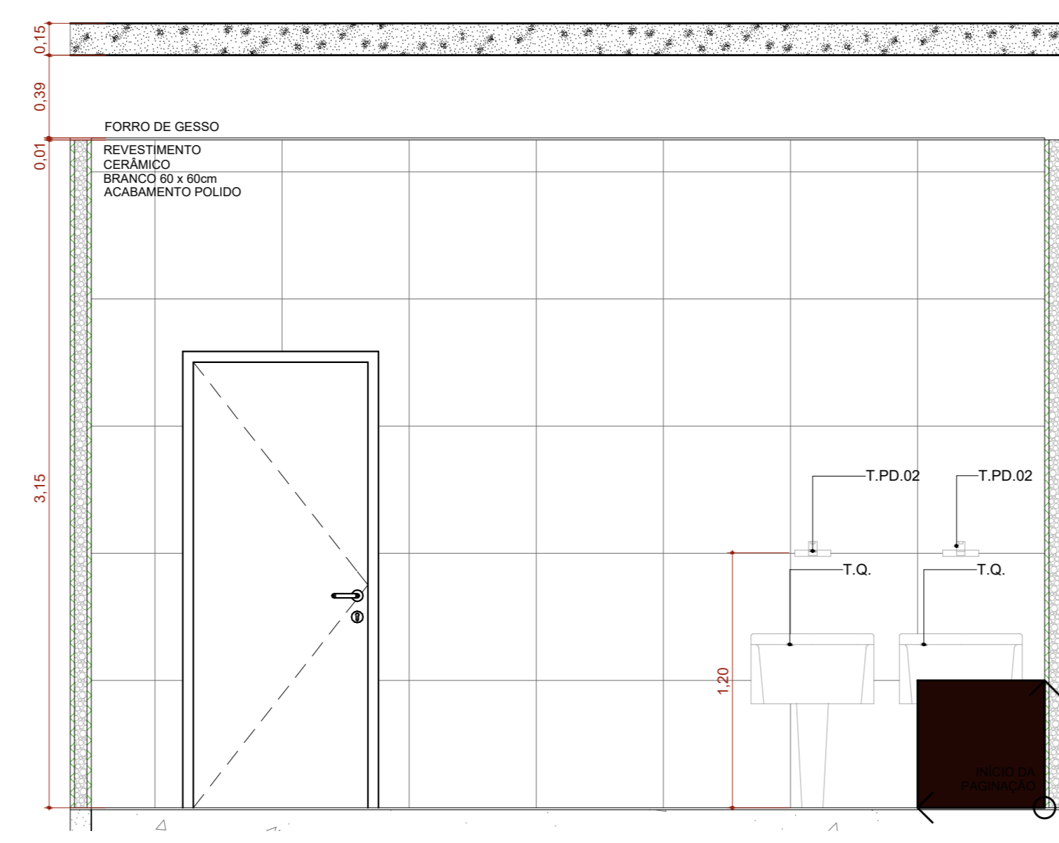
A.M.09 VISTA 02 Escala: 1:25
