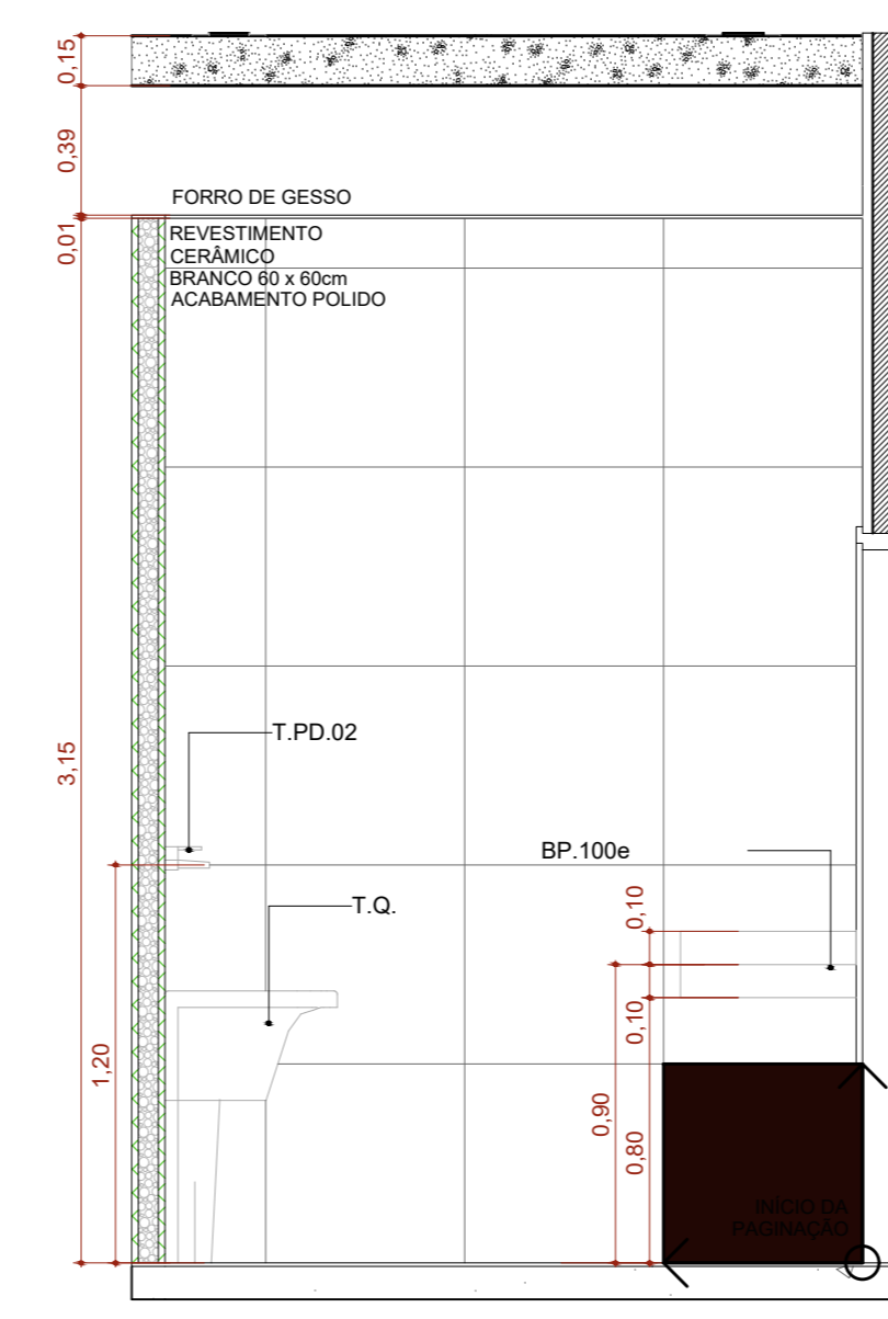
A.M.09 VISTA 03 Escala: 1:25
