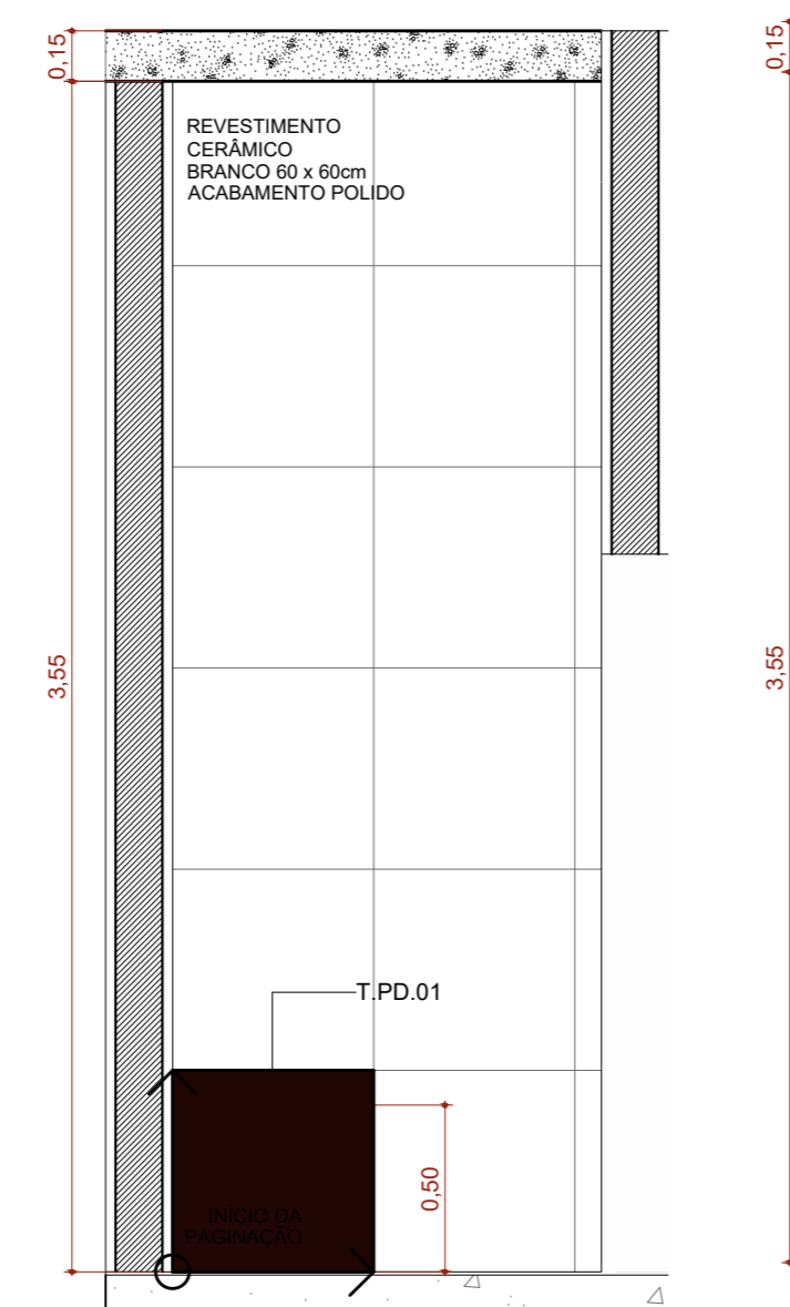
A.M.10 VISTA 03 Escala: 1:25
