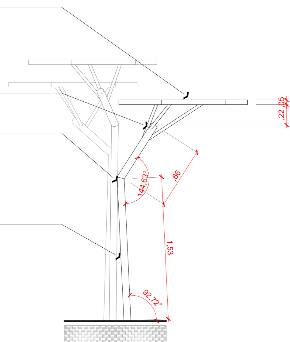
SOMBREIRO - VISTA C ESCALA 1:25
