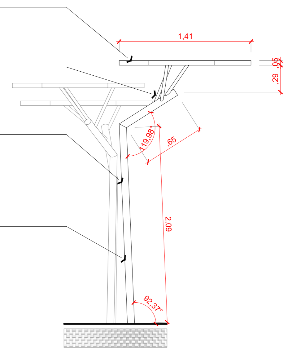
SOMBREIRO - VISTA A ESCALA 1:25
