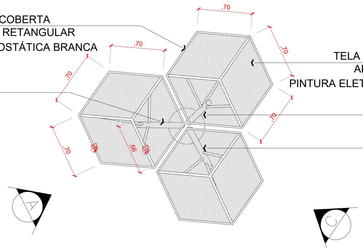
SOMBREIRO - VISTA SUPERIOR ESCALA 1:25
