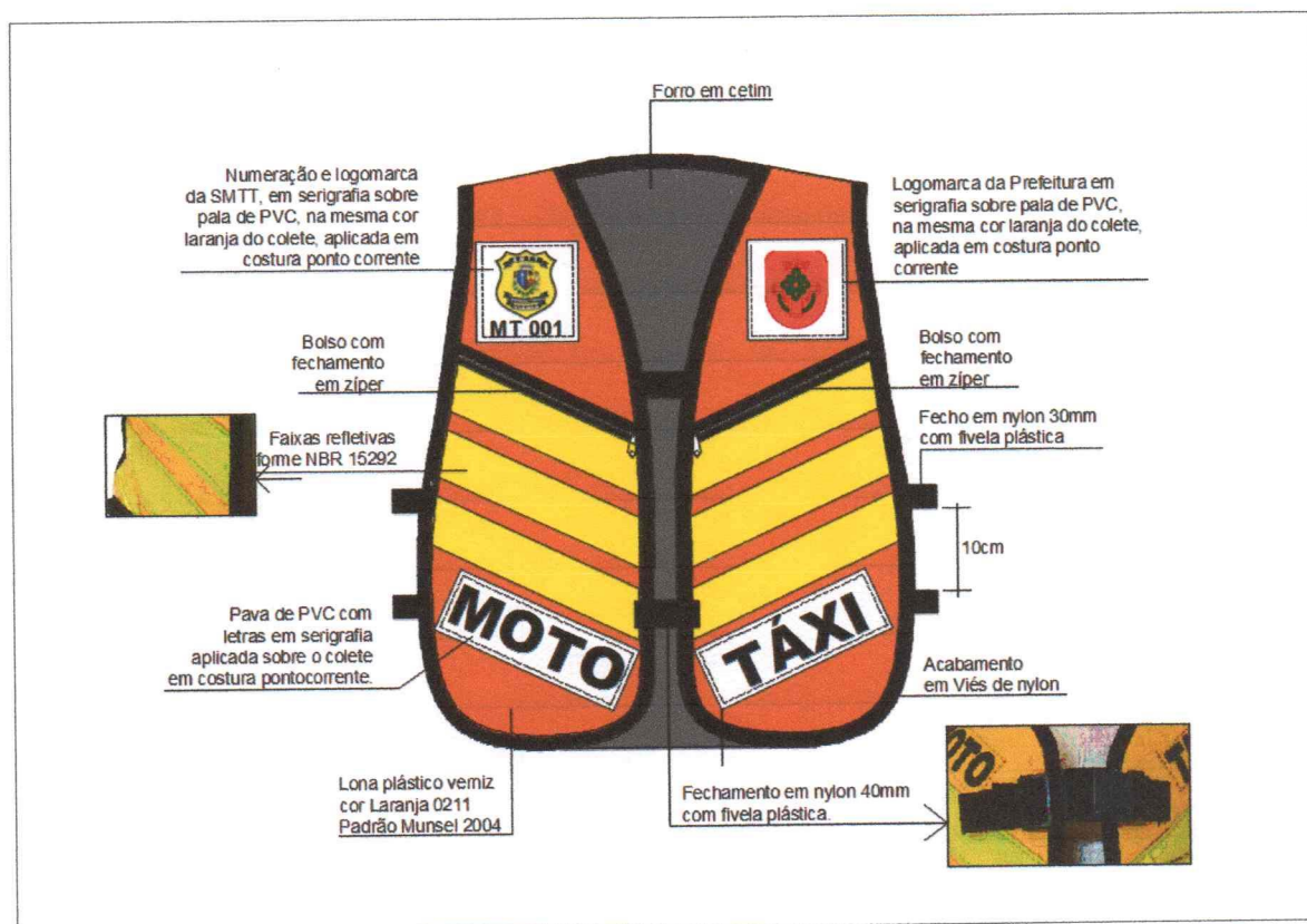
3.13 Detalhe - FRENTE
