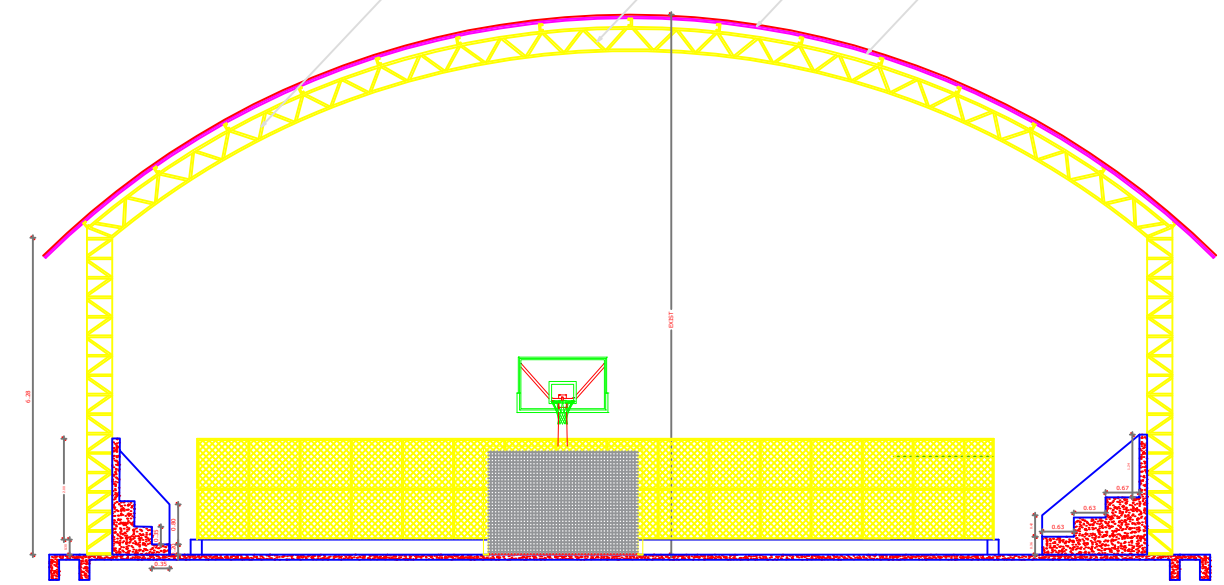
CORTE ESCALA 1:50
