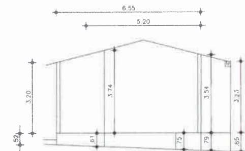
CORTE AA2
