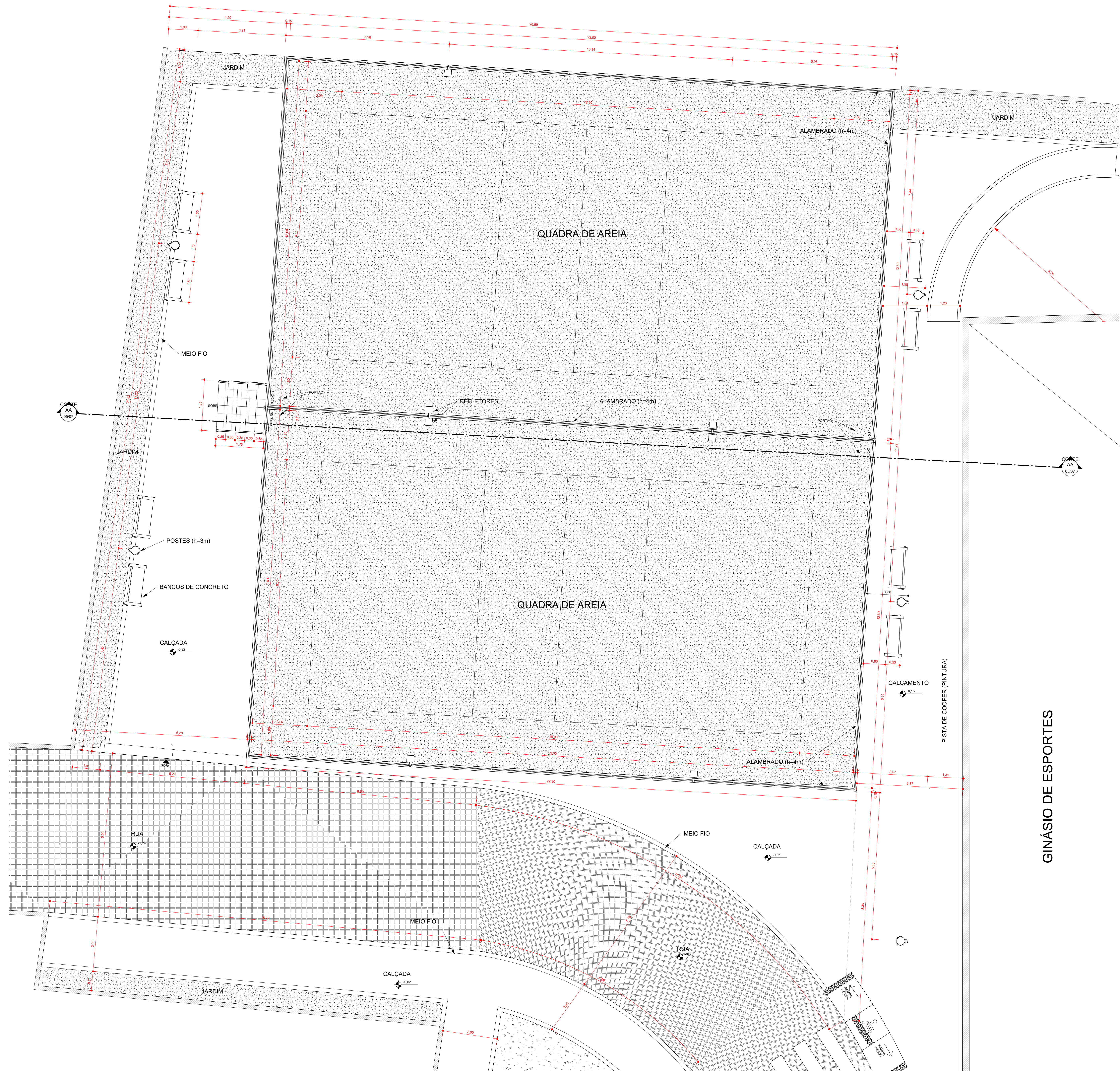
1 IMPLANTAÇÃO QUADRAS ESCALA - 1 : 50
