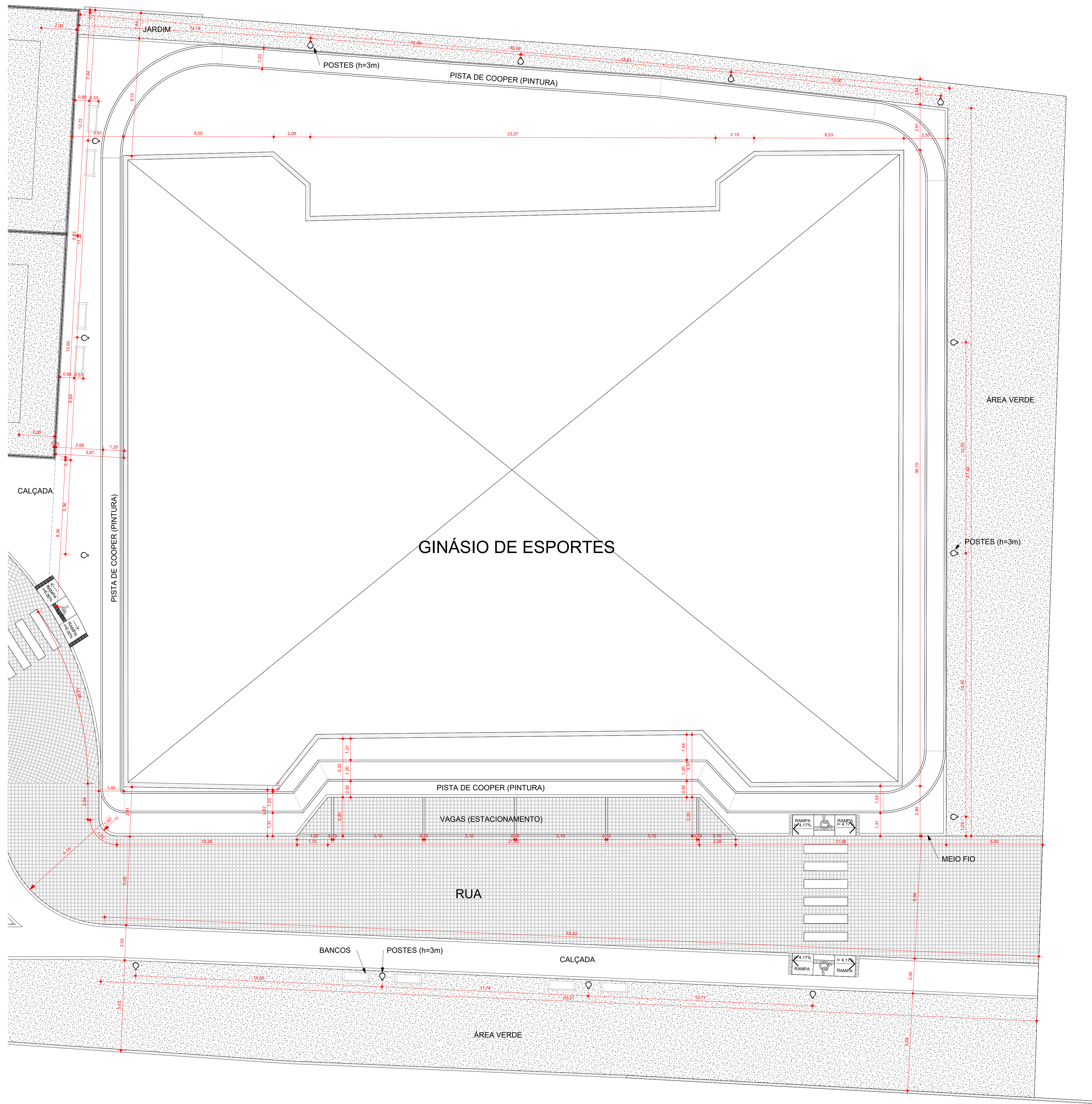
1 IMPLANTAÇÃO GINÁSIO ESCALA - 1 : 100
