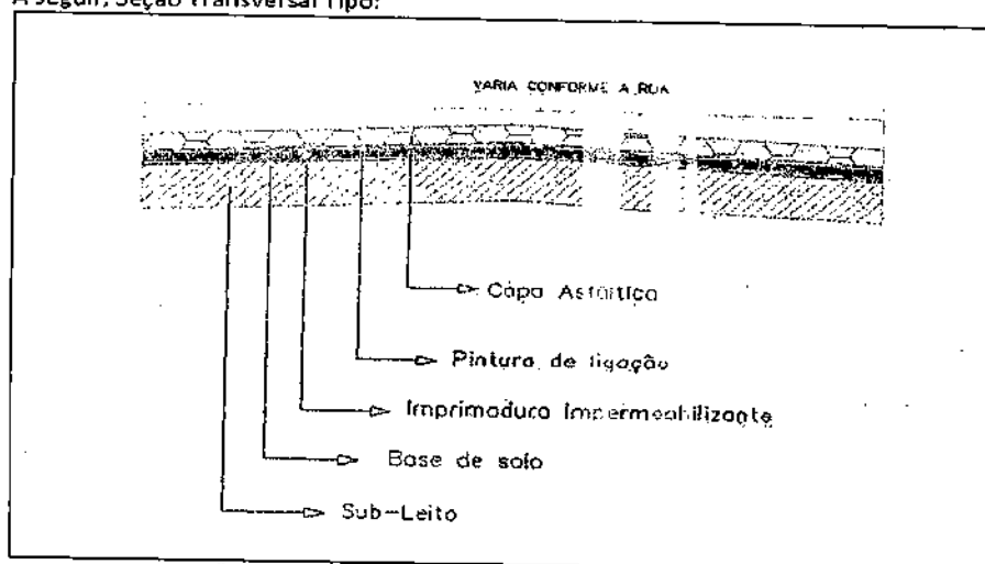
IMAGEM 39 – SEÇÃO TRANSVERSAL TIPO
