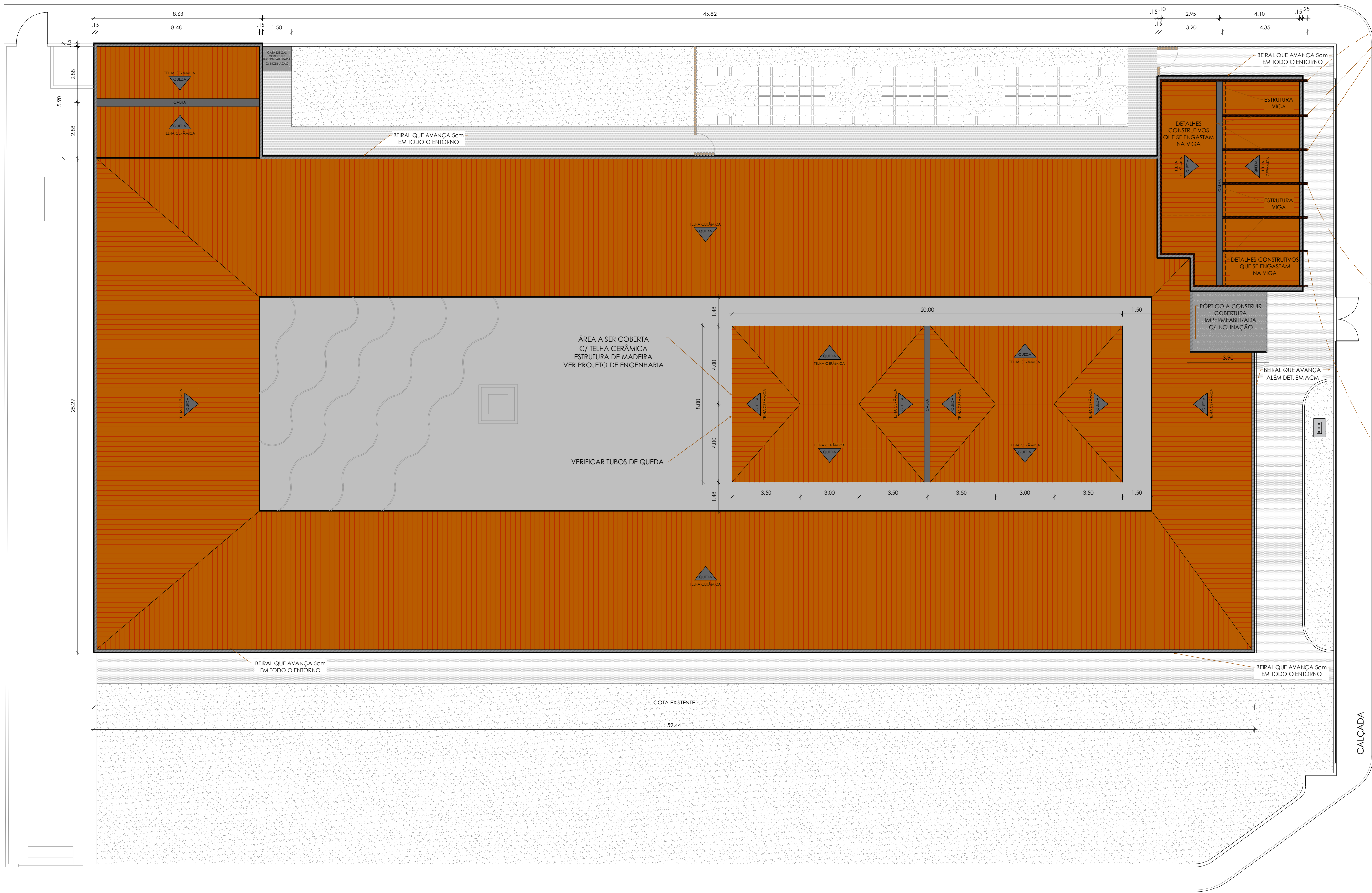
03 PLANTA DE COBERTURA ESCALA 1/125
