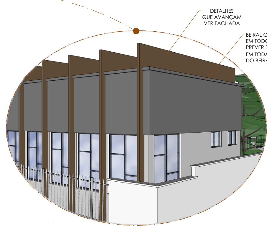
03.1 DETALHES - FACHADA/COBERTURA ESCALA 1/125
