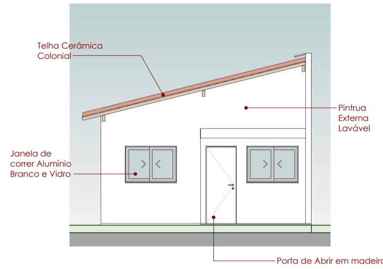
2 Fachada Frente 1 : 100
