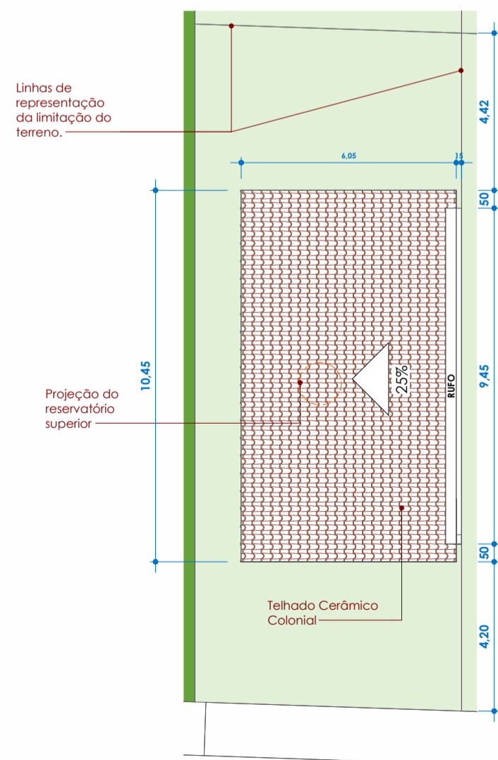
5 Planta de Cobertura Casa 2 1 : 150
