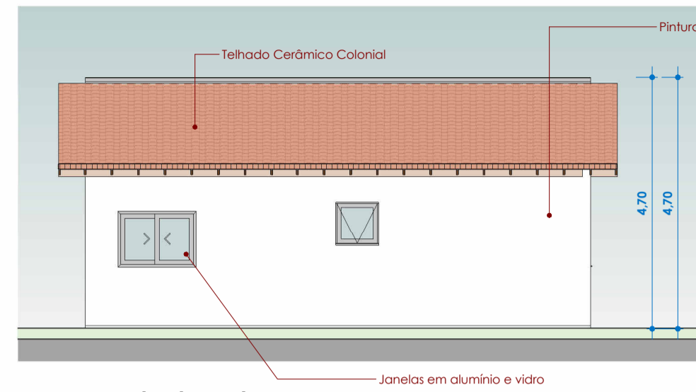
3 Fachada Leste 1 : 100
