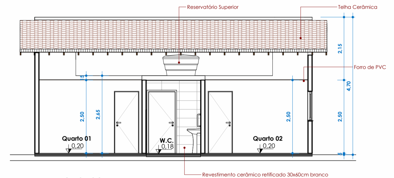
7 Corte 04 1 : 75
