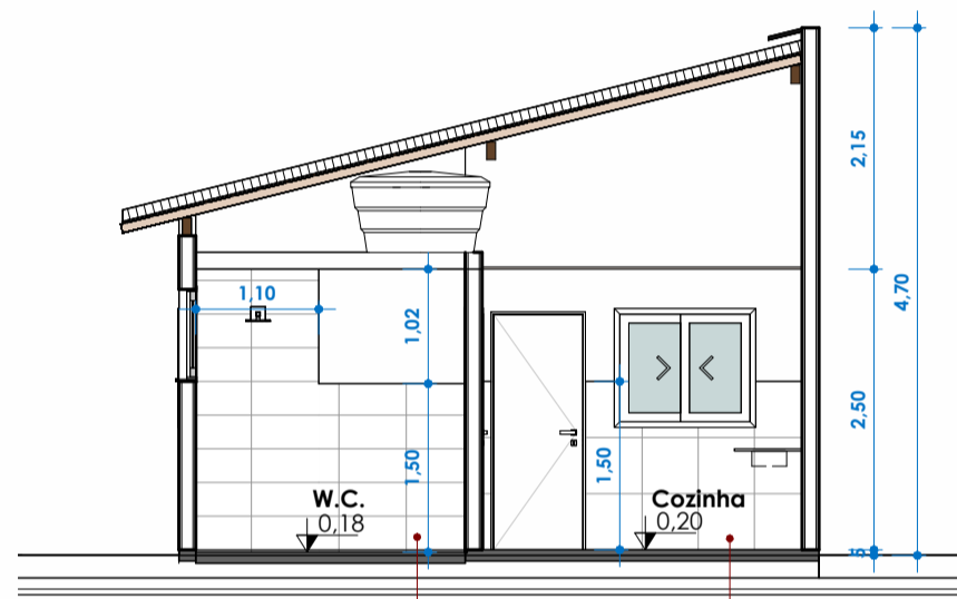
6 Corte 03 1 : 75
