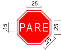
R-1 PARADA OBRIGATÓRIA
