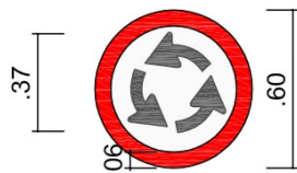
R-33 SENTIDO DE CIRCULAÇÃO NA ROTATÓRIA
