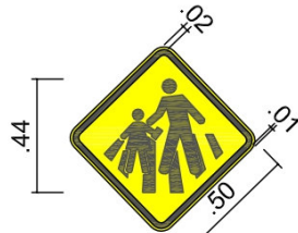
A-33b PASSAGEM SINALIZADA DE ESCOLARES
