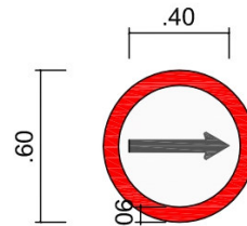
R-24a SENTIDO DE CIRCULAÇÃO DA VIA
