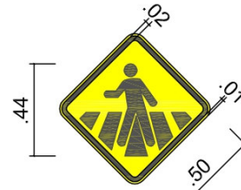
A-32b PASSAGEM SINALIZADA DE PEDESTRE
