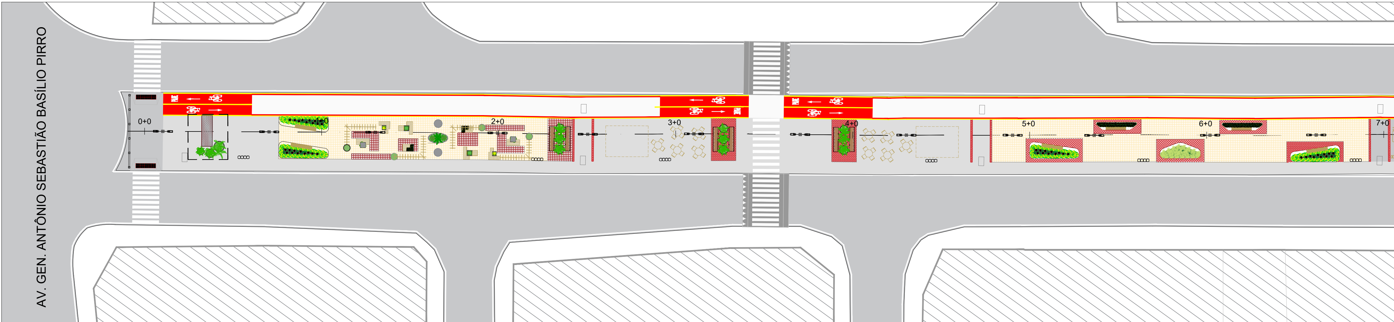
URBANIZAÇÃO DA AV. CANAL DO GUAXINIM - PLANTA DE PAGINAÇÃO DE PISO TRECHO 01 - EST. 0+0 ATÉ 7+0 ESC. 1: 250
