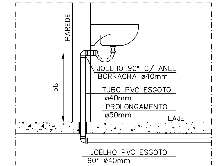
DETALHE LAVATÓRIO - CORTE (CE) SEM ESCALA
