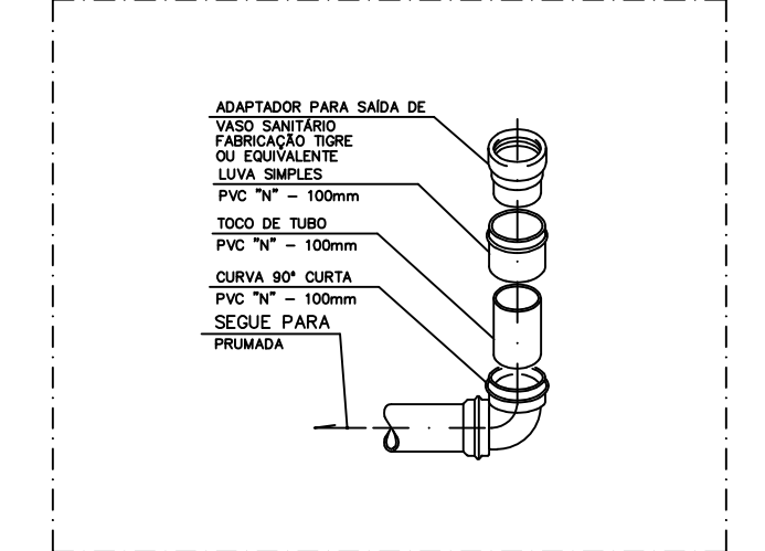
DETALHE MONTAGEM DE VEDAÇÃO SEM ESCALA
