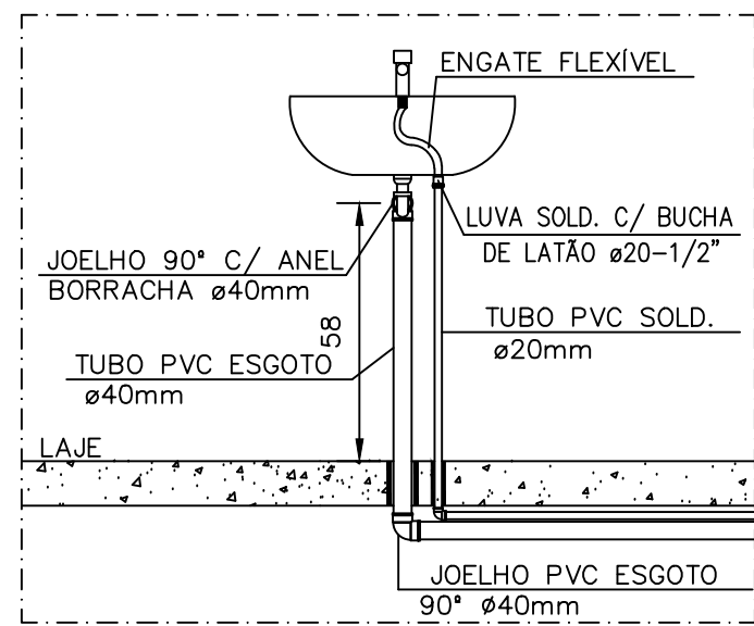
DETALHE LAVATÓRIO - VISTA (CE) SEM ESCALA
