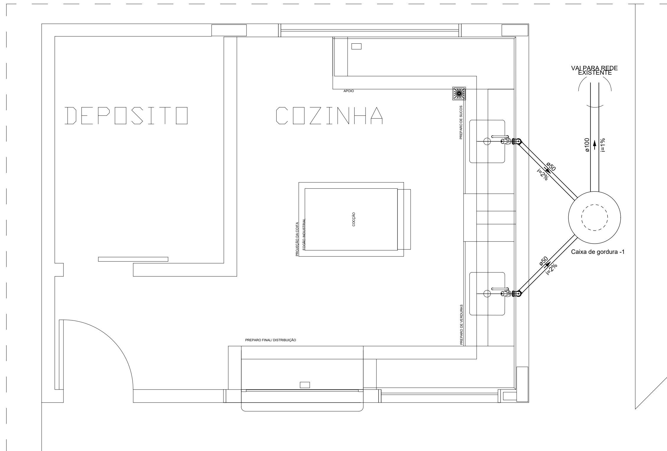
DETALHE SAN-2 1:25
