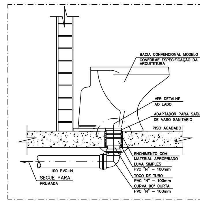
DETALHE LIGAÇÃO VASO SANITÁRIO SEM ESCALA
