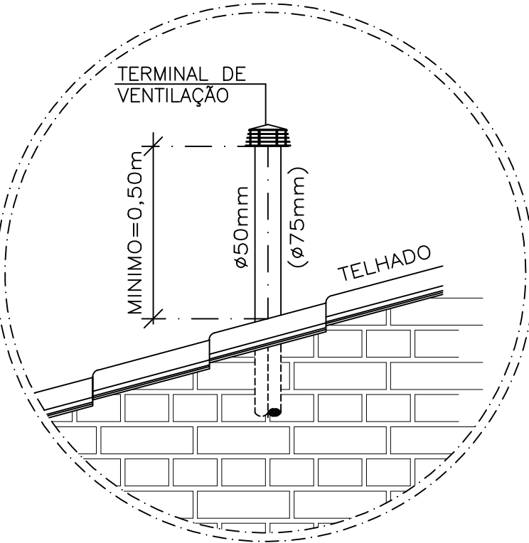
DETALHE EXTREMIDADE COLUNA DE VENTILAÇÃO - VISTA SEM ESCALA
