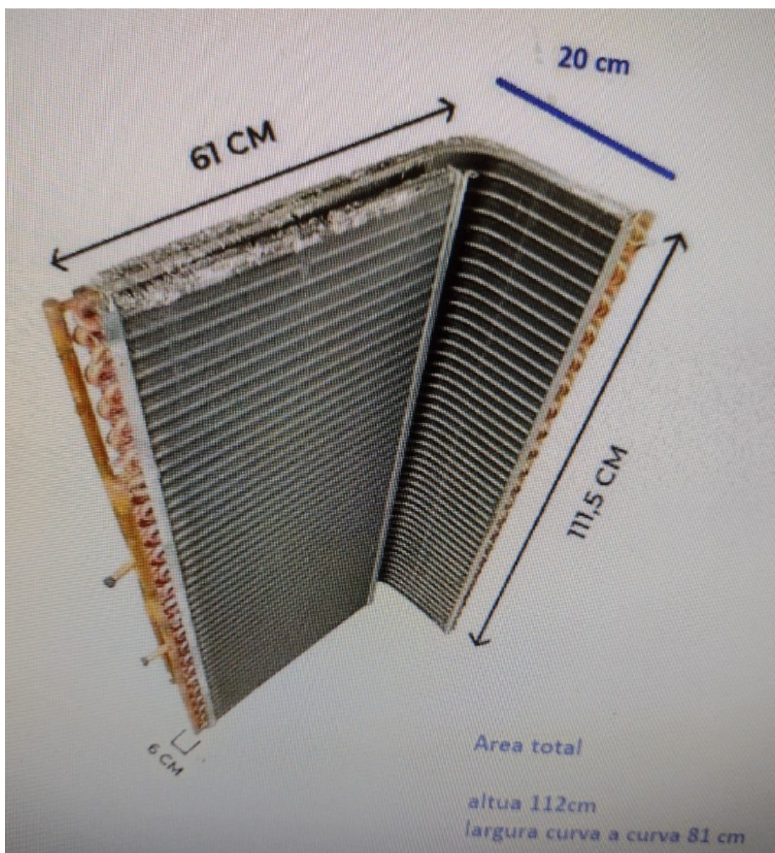
Figura 1: Foto da serpentina a ser adquirida.
