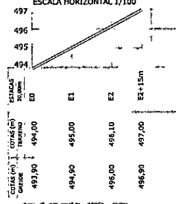
PERFIL LONGITUDINAL; TRAVESSA NELSON FERREIRA 01; EXTENSÃO=55,00 m; LARGURA=6,00 m ESCALA VERTICAL 1/1000 ESCALA HORIZONTAL 1/100
