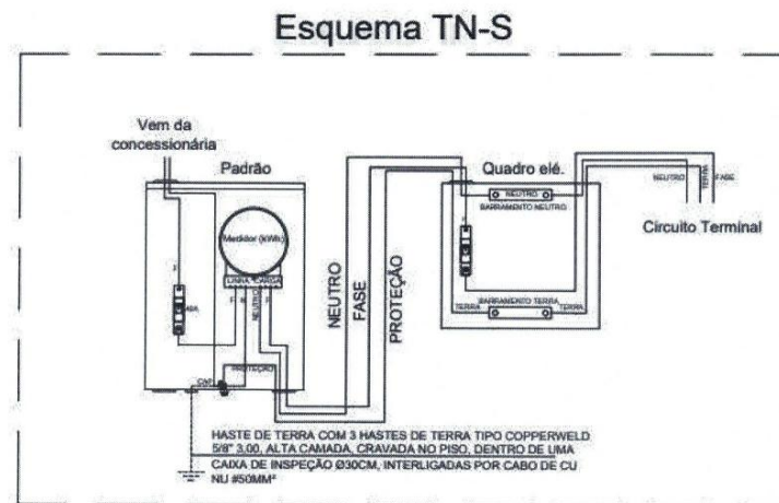
Figura 02– Esquema TN-S_Detalhe da instalação do medidor de energia e do Quadro de distribuição Sistema Monofásico
