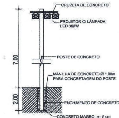
Figura 03– Vista frontal do sistema de iluminação em LED
