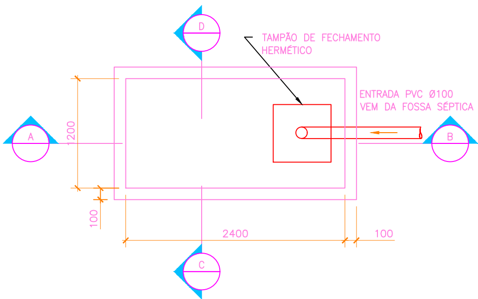
SUMIDOURO PRISMÁTICO RETANGULAR-PLANTA
