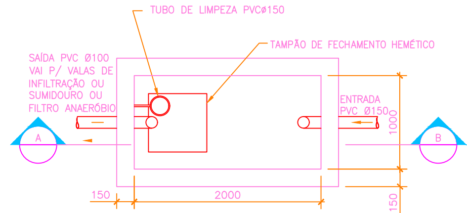
TANQUE SÉPTICO PRISMÁTICO RETANGULAR-PLANTA
