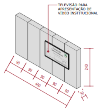
DETALHE PAINEL EM MDF S18 ESCALA - 1:50
