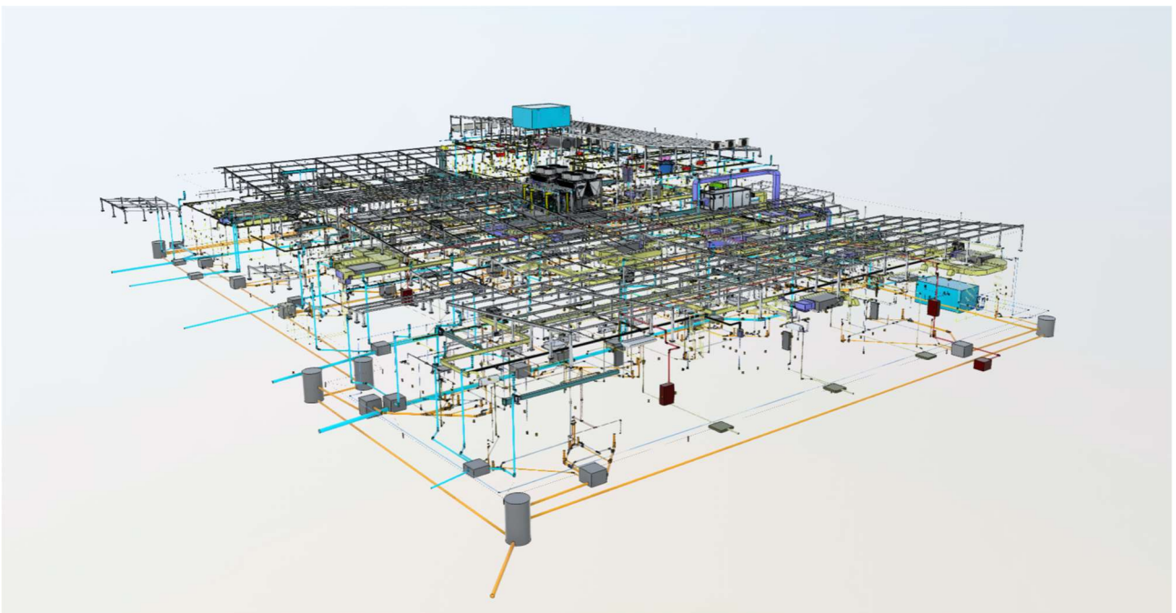
Figura 2: Modelo Instalações prediais
