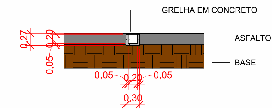
Corte - Grelha
