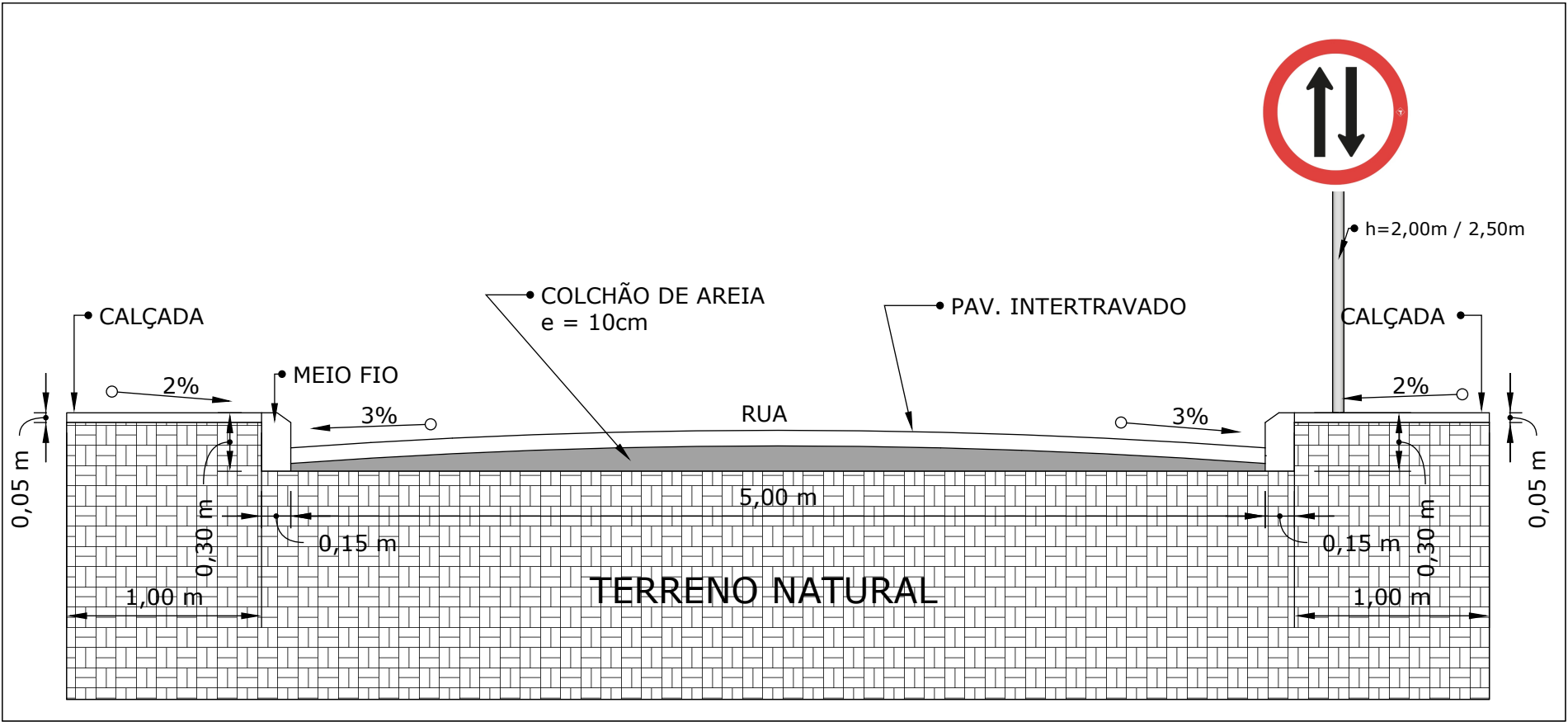
1 SEÇÃO TRANSVERSAL 1:50
