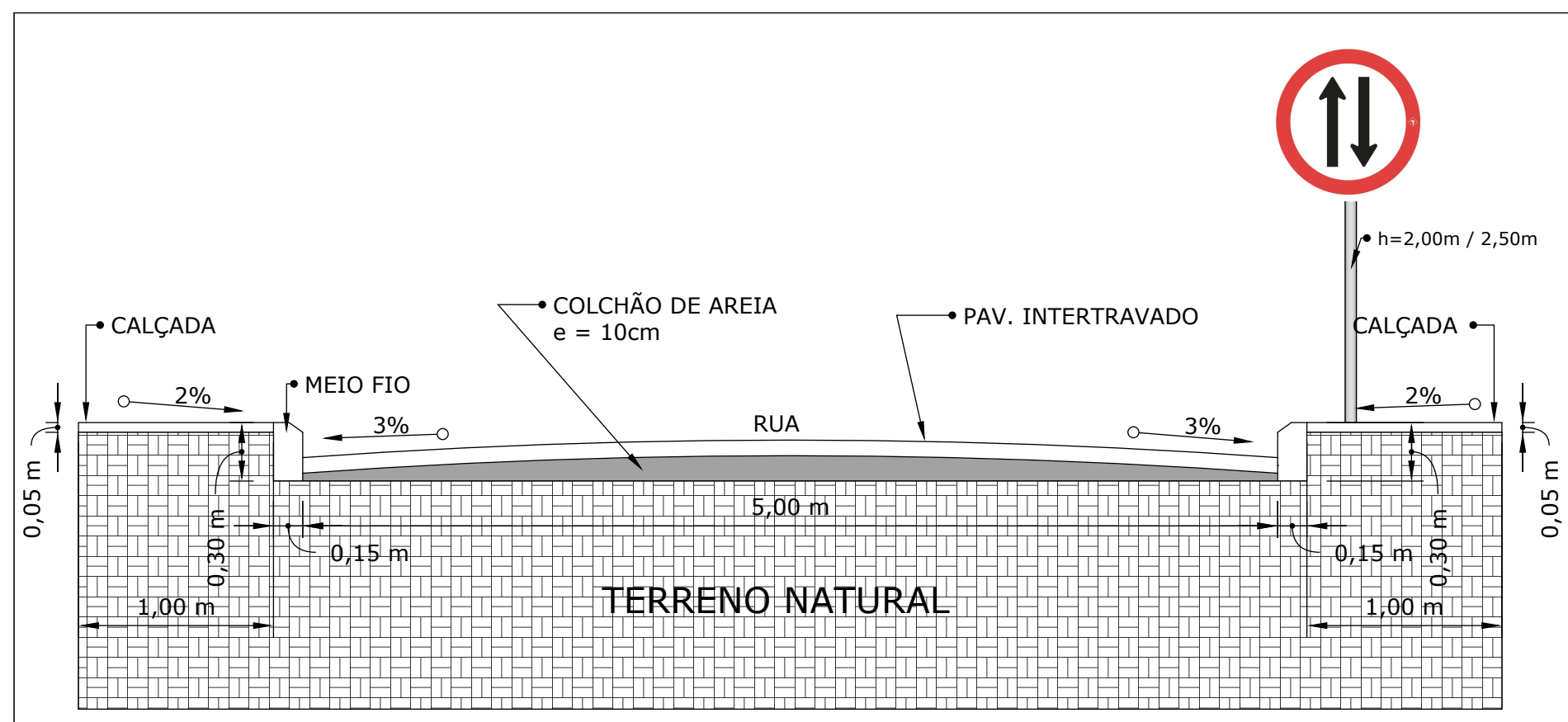
1 SEÇÃO TRANSVERSAL
