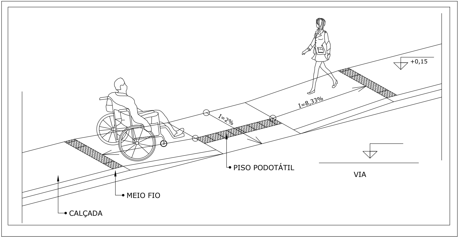
4 RAMPA EM PERSPECTIVA 1:50
