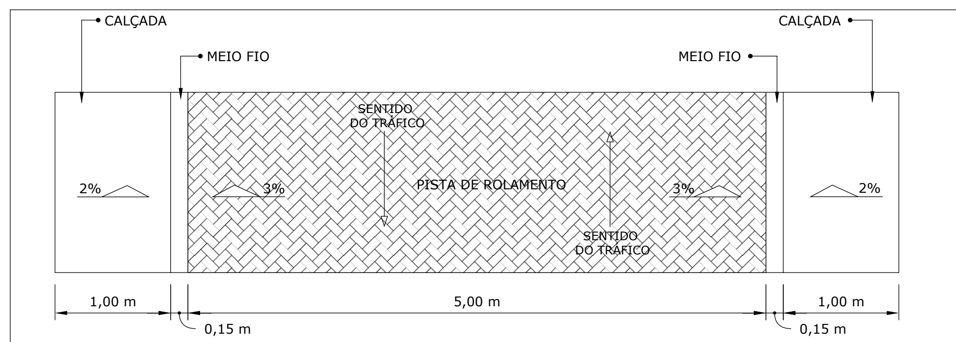
3 DIAGRAMAÇÃO DE PISTA DE ROLAMENTO
