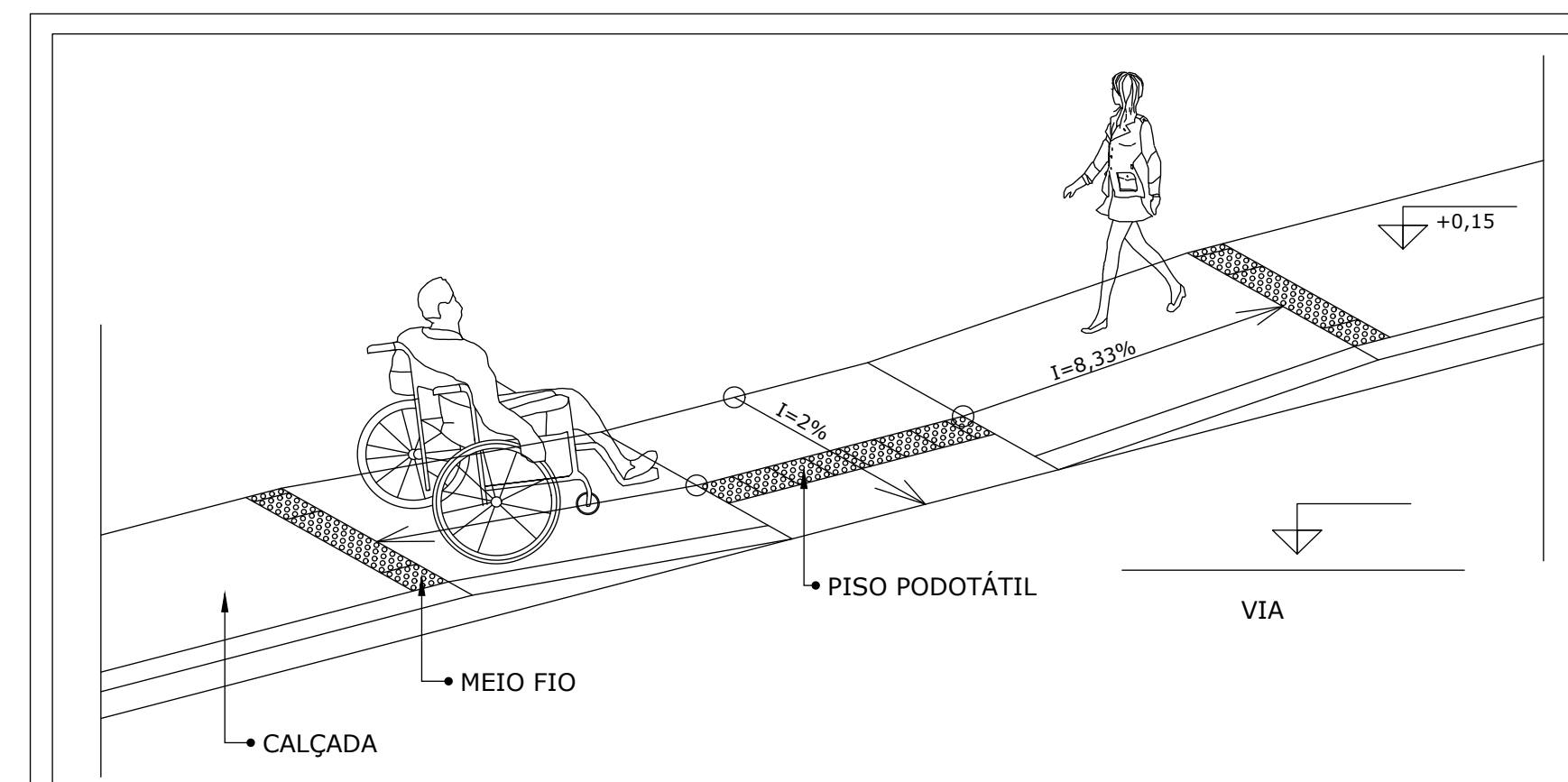
4 RAMPA EM PERSPECTIVA
