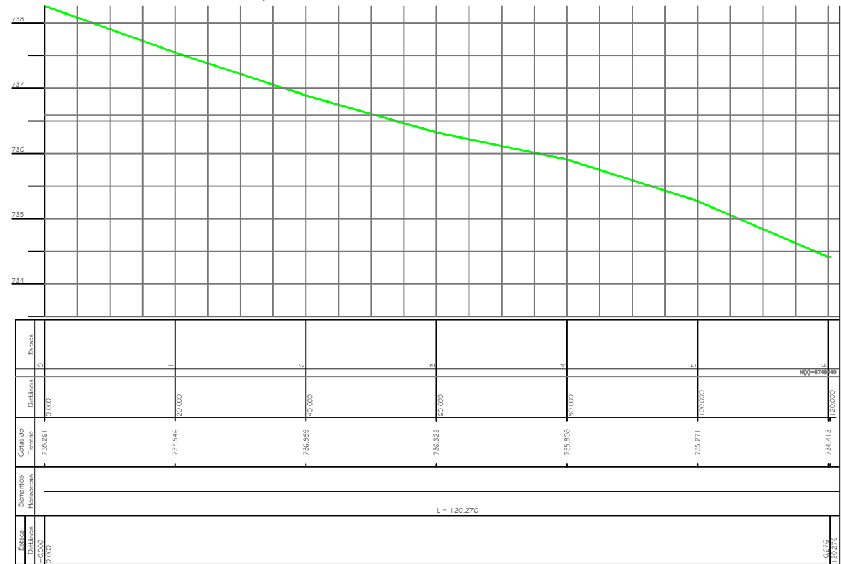
RUA CAMPUS AVANÇADO PERFIL LONGITUDINAL ESCALA - H=1/500;V=1/50
