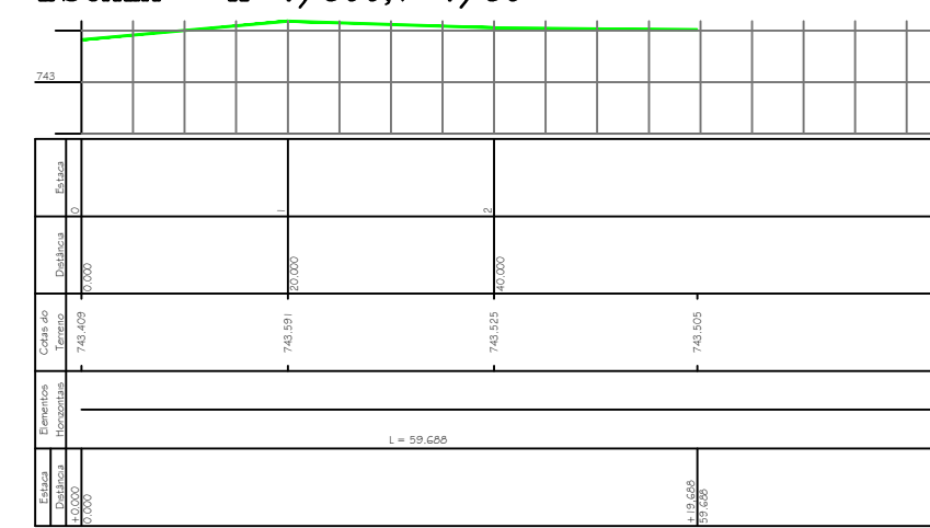
RUA EURICO GASPAR DUTRA PERFIL LONGITUDINAL ESCALA - H=1/500;V=1/50
