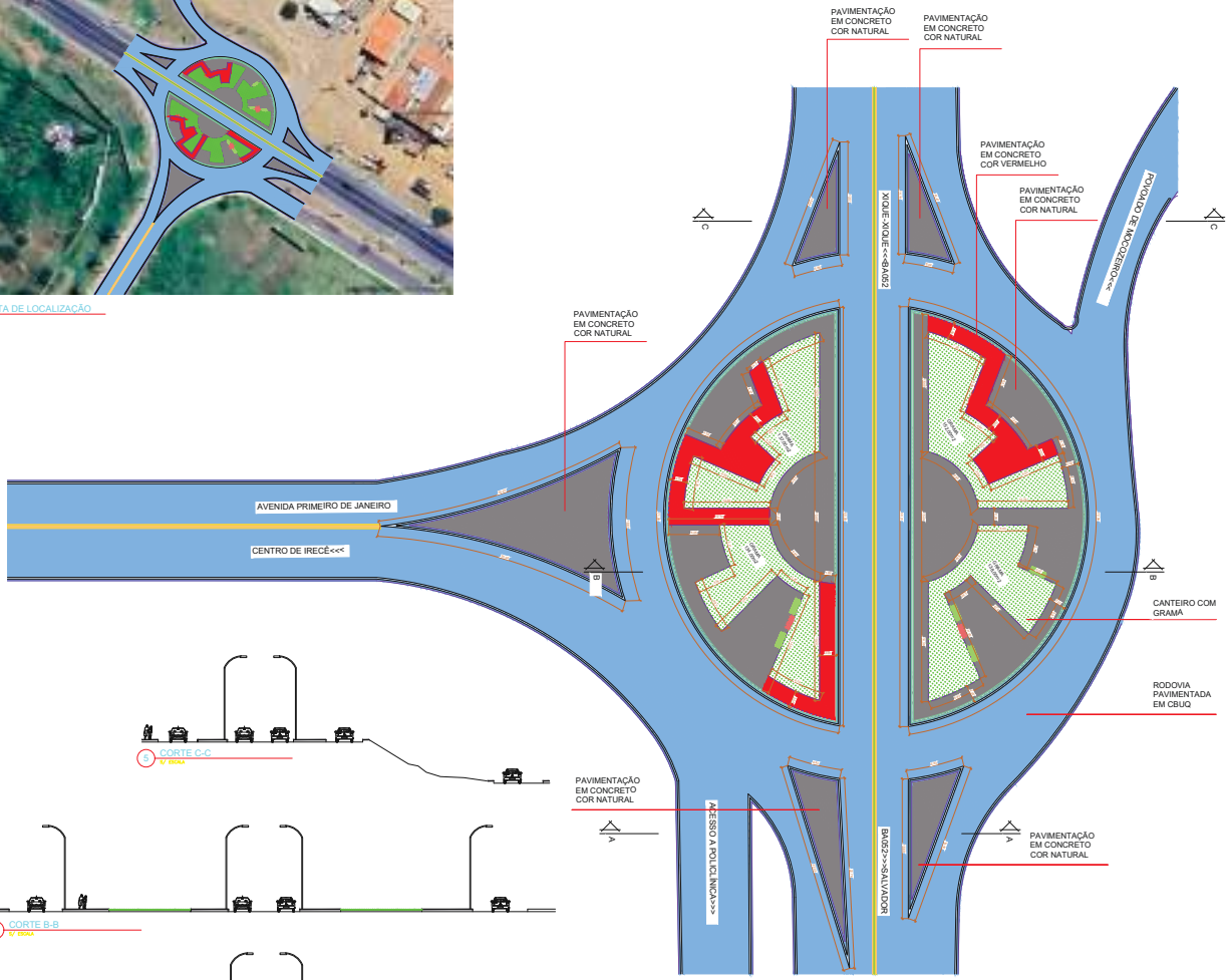
2 PLANTA BAIXA V. ESCALA
