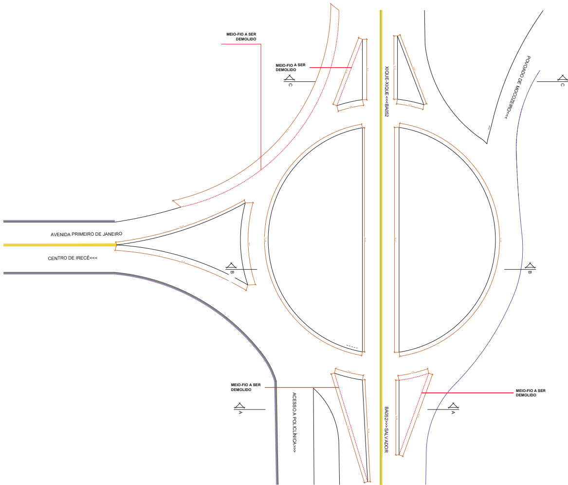
1 PLANTA DE DEMOLIÇÃO 1/5000
