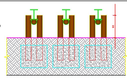
VISTA FRONTAL ESCALA 1/25
