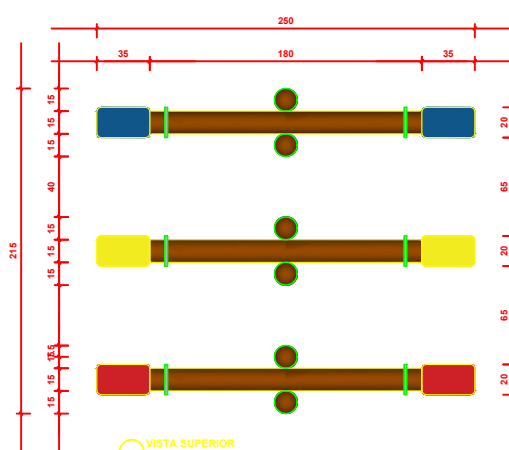
VISTA SUPERIOR ESCALA 1/25
