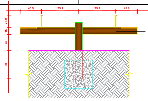
VISTA LATERAL ESCALA 1/25
