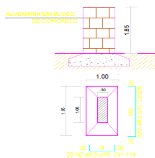
TOTEM 1 3x(1,00x1,85)
