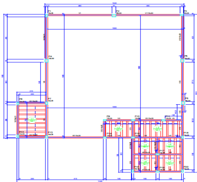
Forma do pavimento Térreo (Nível 300) escala 1:50
