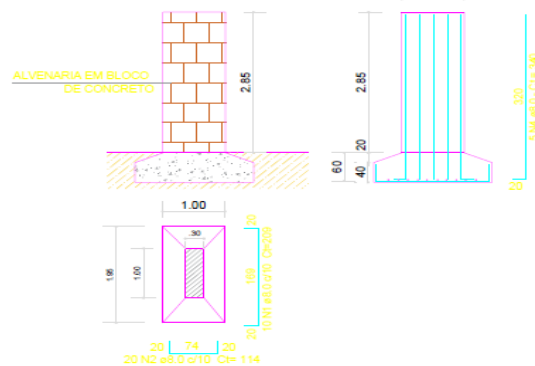
TOTEM 2 3x(1,00x2,85)
