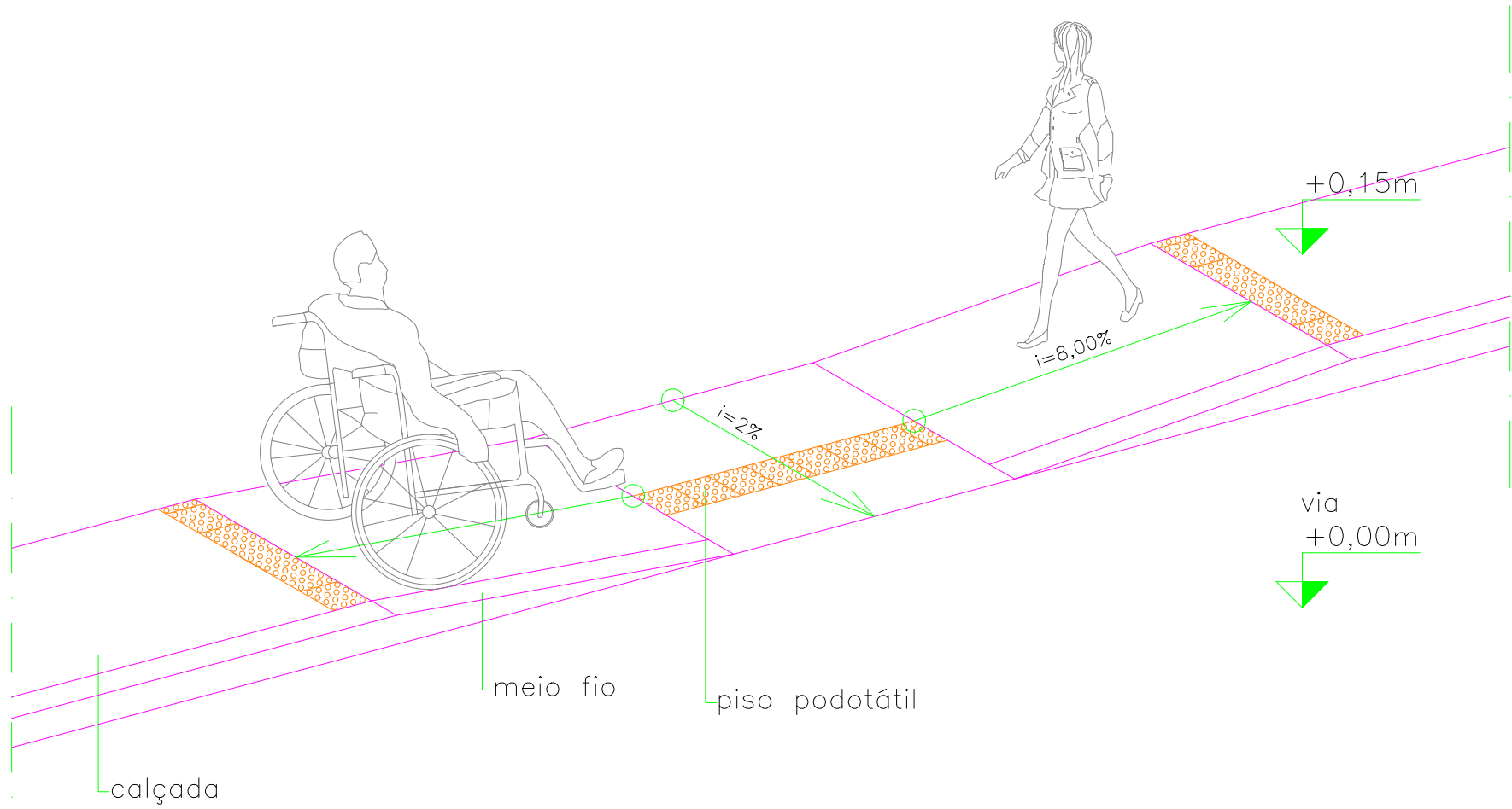
RAMPA EM PERSPECTIVA
