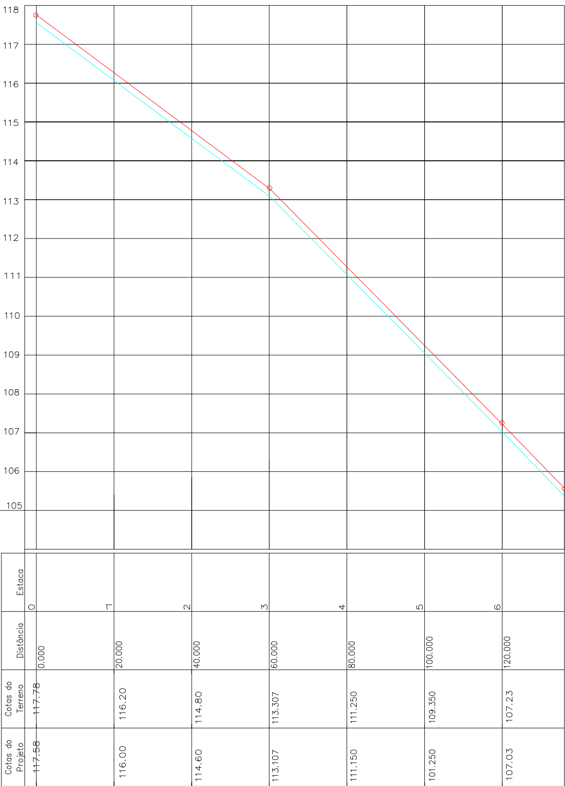
PERFIL LONGITUDINAL DA RUA (A) ESCALAS: H-1:1.000 V-1:100
