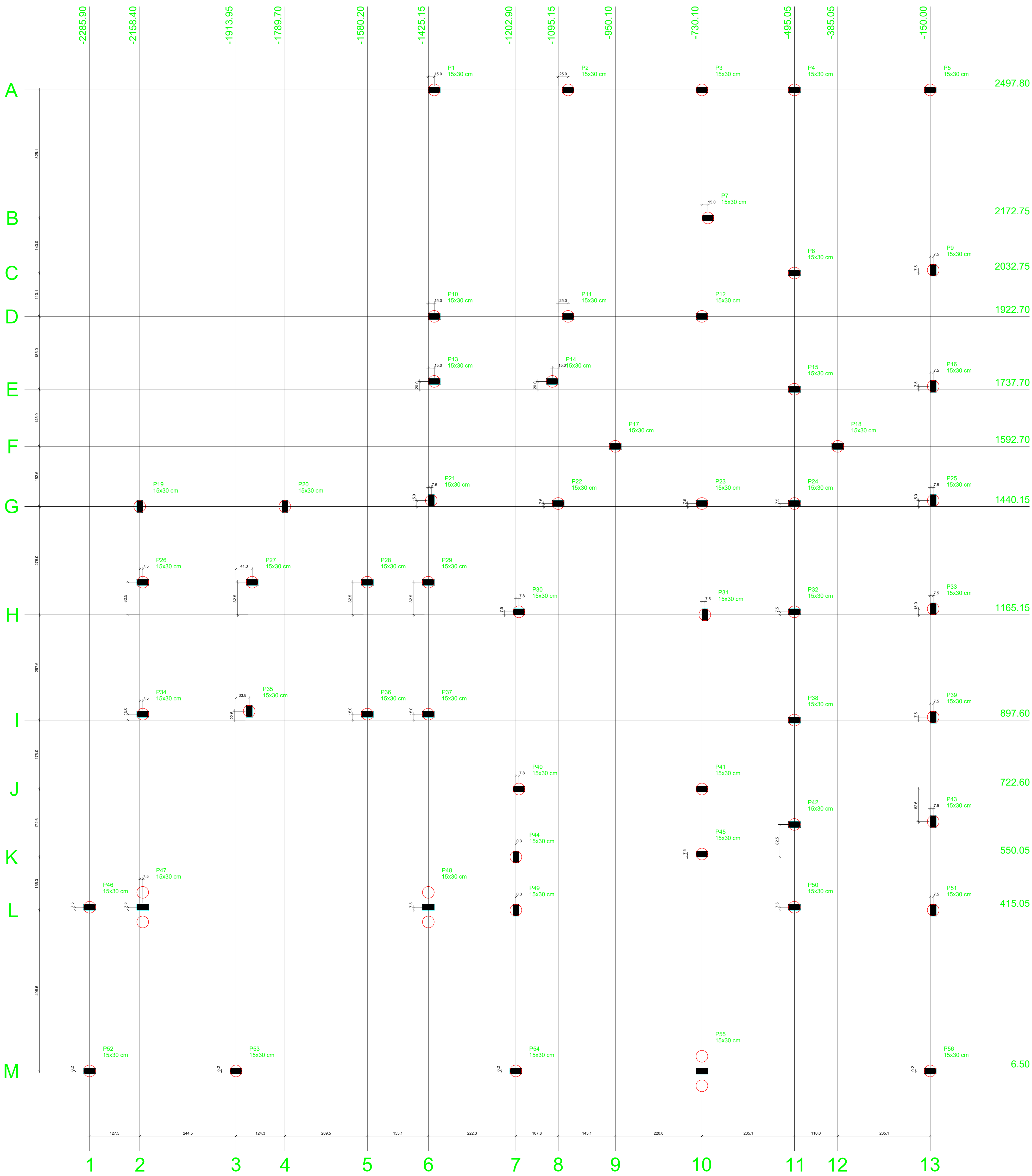
Planta de locação das estacas escala 1:30
