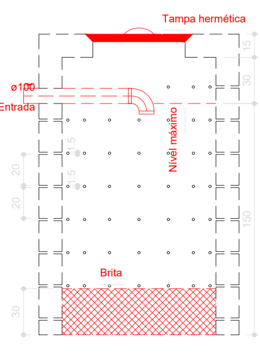
Sumidouro - Pavimento Térreo Corte 1 - ESC. 1:25
