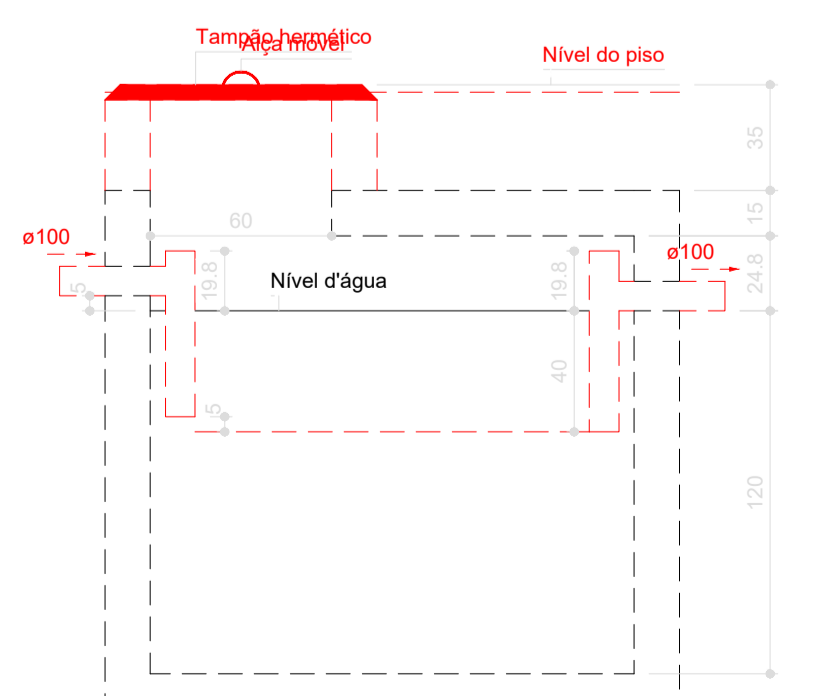
Tanque séptico - Pavimento Térreo Corte 1 - ESC. 1:25
