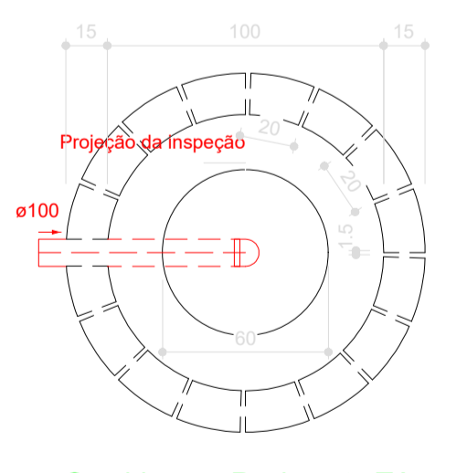
Sumidouro - Pavimento Térreo Planta baixa - ESC. 1:25
