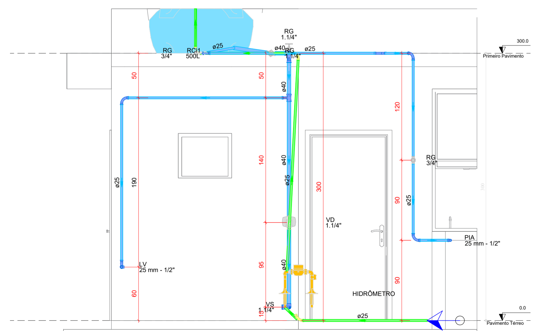
Detalhe HID-3 Escala 1:25
