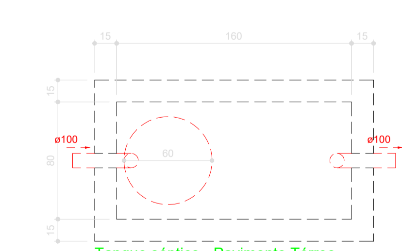
Tanque séptico - Pavimento Térreo Planta baixa - ESC. 1:25
