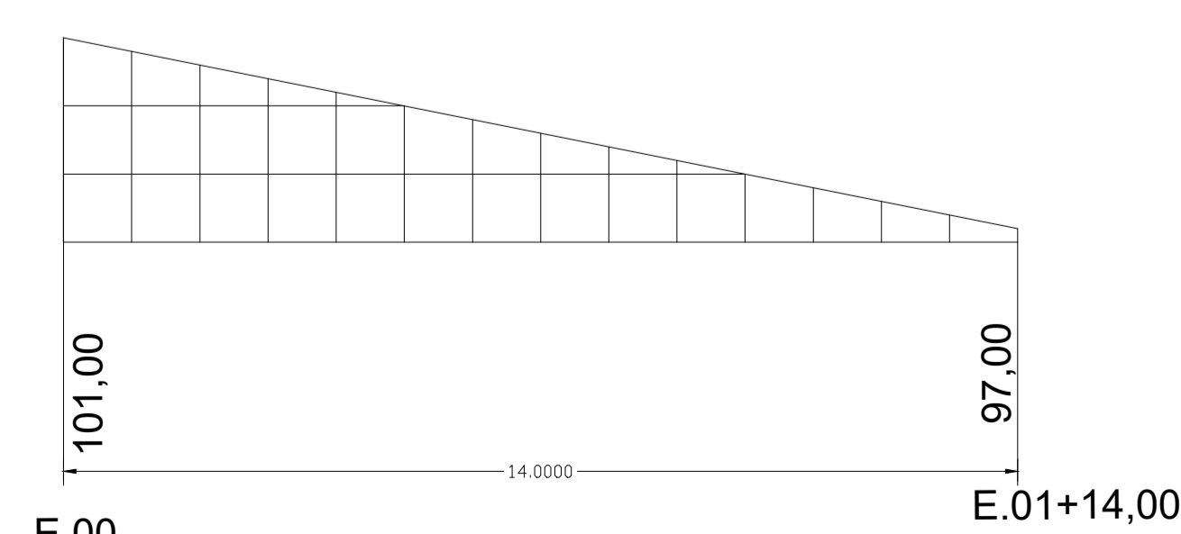
Corte A-B
