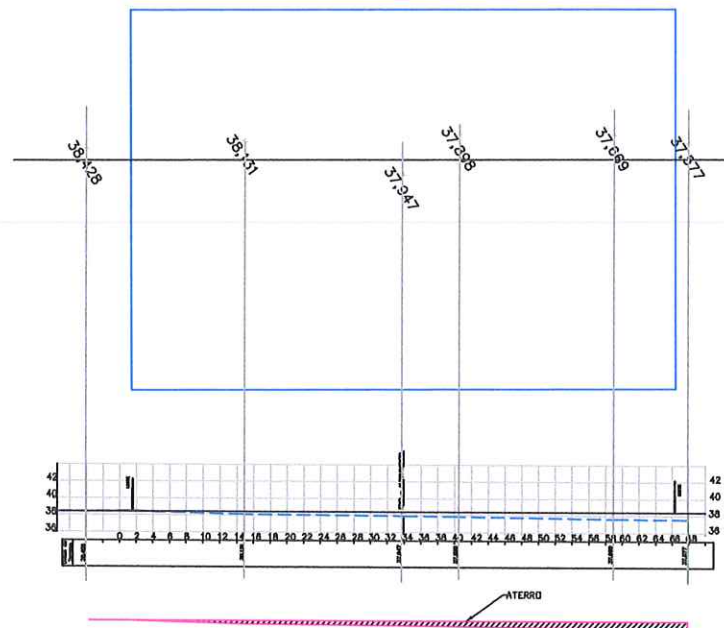
PERFIL LONGITUDINAL
