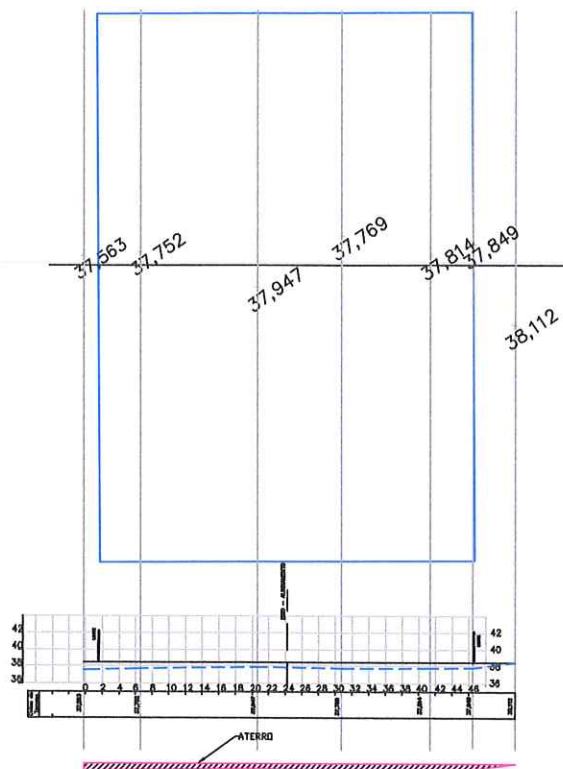
PERFIL TRANSVERSAL
