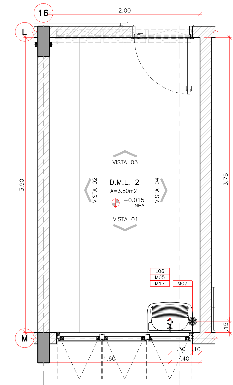
02 UNIDADE DE PRONTO ATENDIMENTO – PORTE 1 D.M.L. 2 ESCALA: 1:25
