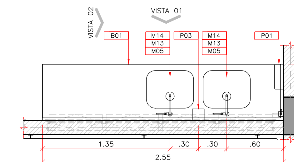
04 UNIDADE DE PRONTO ATENDIMENTO – PORTE 1 BANCADA 07 ESCALA: 1:25
