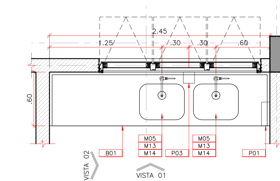
03 UNIDADE DE PRONTO ATENDIMENTO – PORTE 1 BANCADA 06 ESCALA: 1:25
