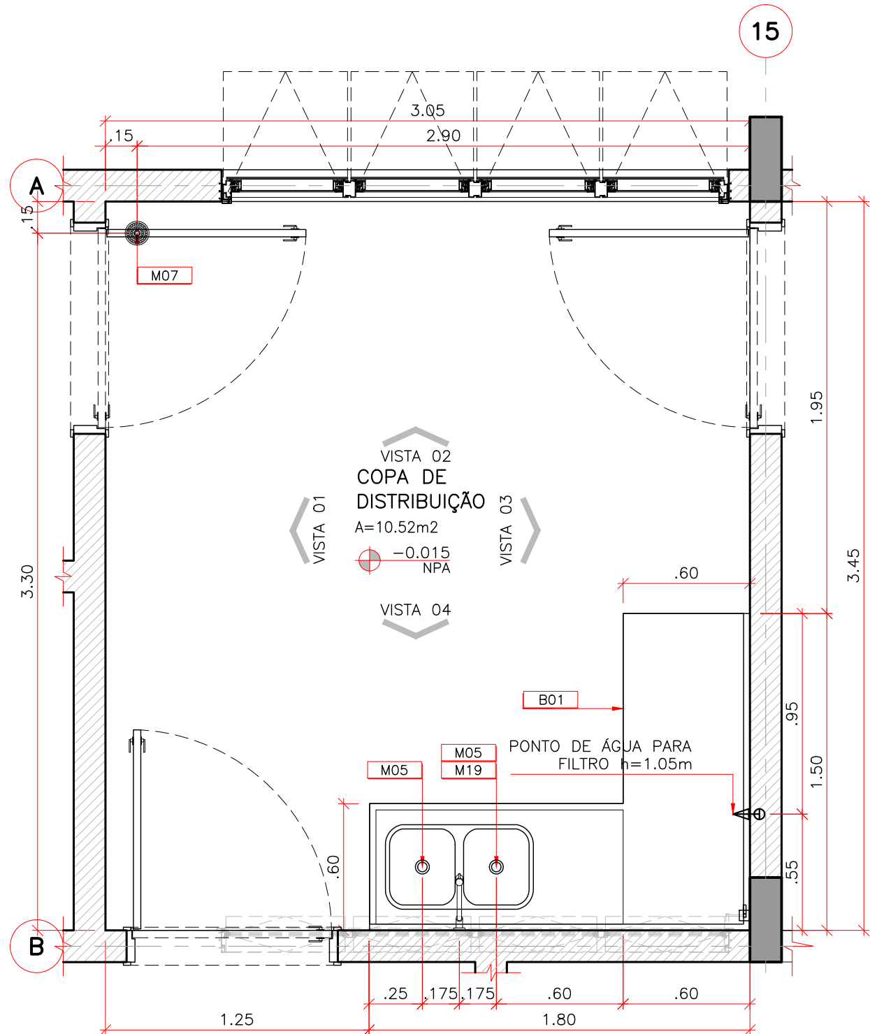
01 UNIDADE DE PRONTO ATENDIMENTO – PORTE 1 COPA DE DISTRIBUIÇÃO ESCALA: 1:25
