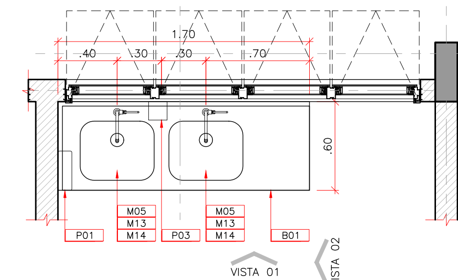
03 UNIDADE DE PRONTO ATENDIMENTO – PORTE 1 BANCADA 01 ESCALA: 1:25
