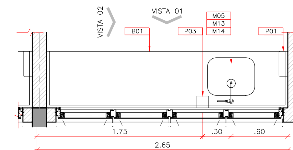
04 UNIDADE DE PRONTO ATENDIMENTO – PORTE 1 BANCADA 02 ESCALA: 1:25
