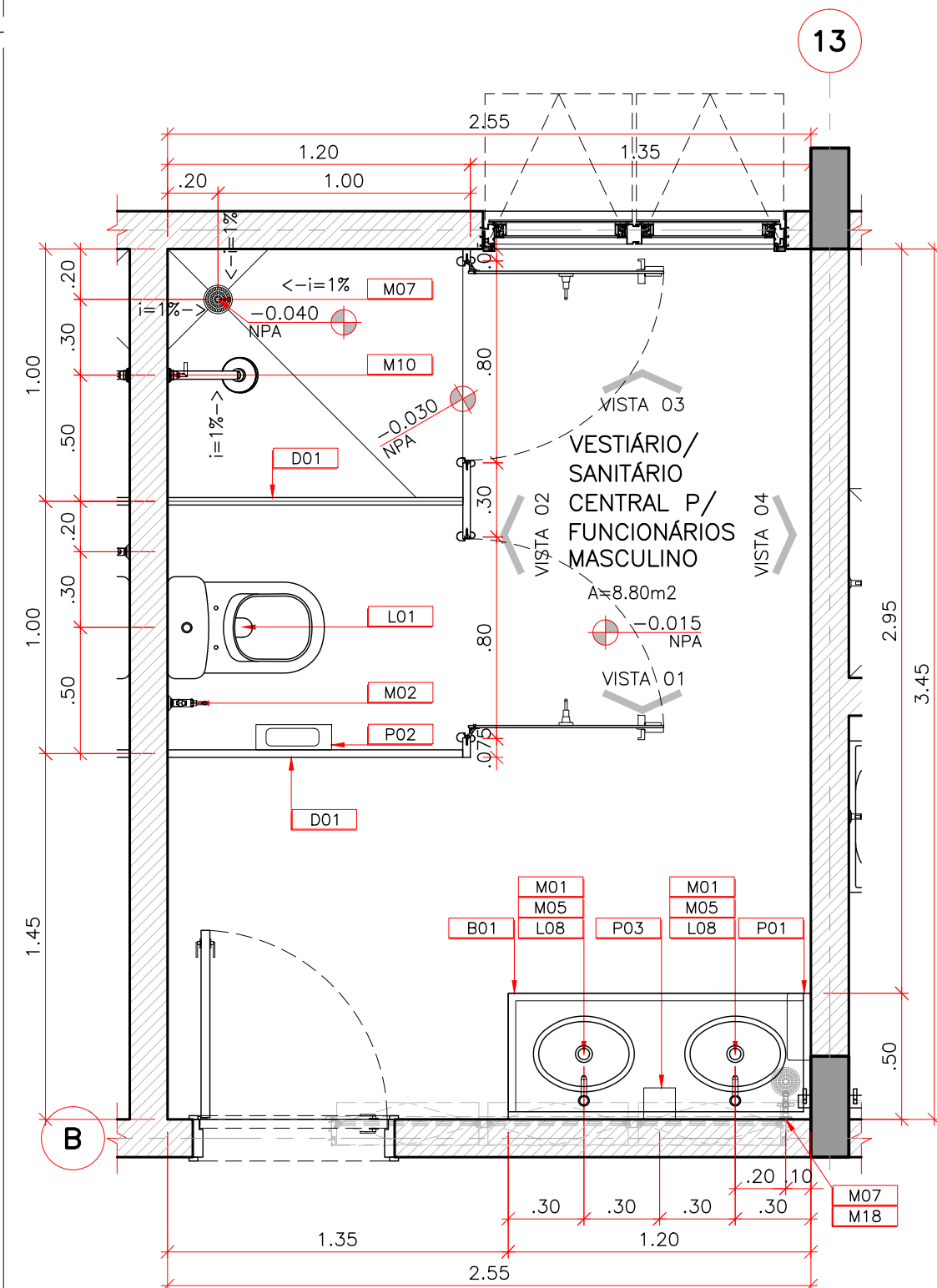
02 UNIDADE DE PRONTO ATENDIMENTO – PORTE 1 VESTIÁRIO/ SANITÁRIO P/ FUNC. MASCULINO ESCALA: 1:25
