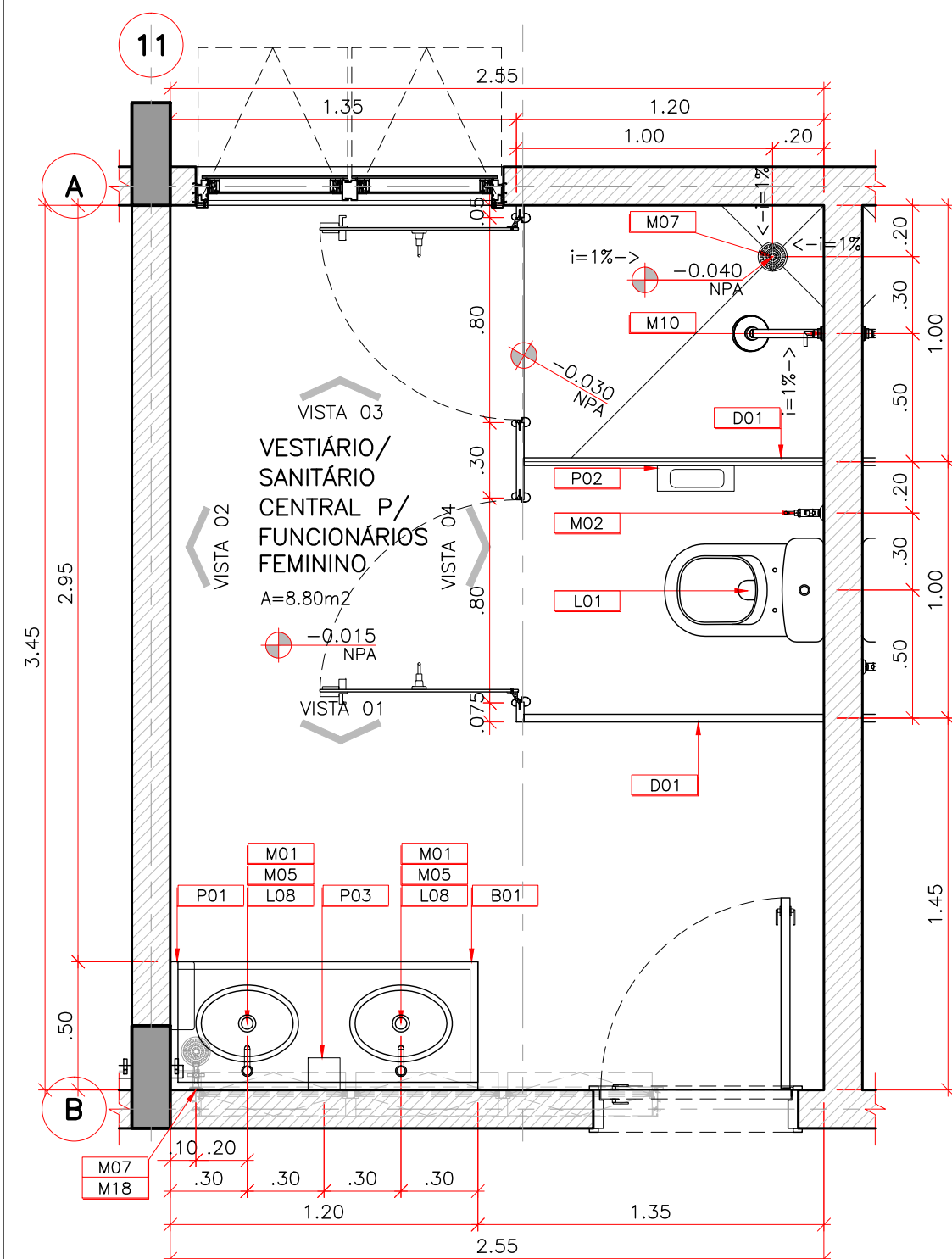
01 UNIDADE DE PRONTO ATENDIMENTO – PORTE 1 VESTIÁRIO/ SANITÁRIO P/ FUNC. FEMININO ESCALA: 1:25
