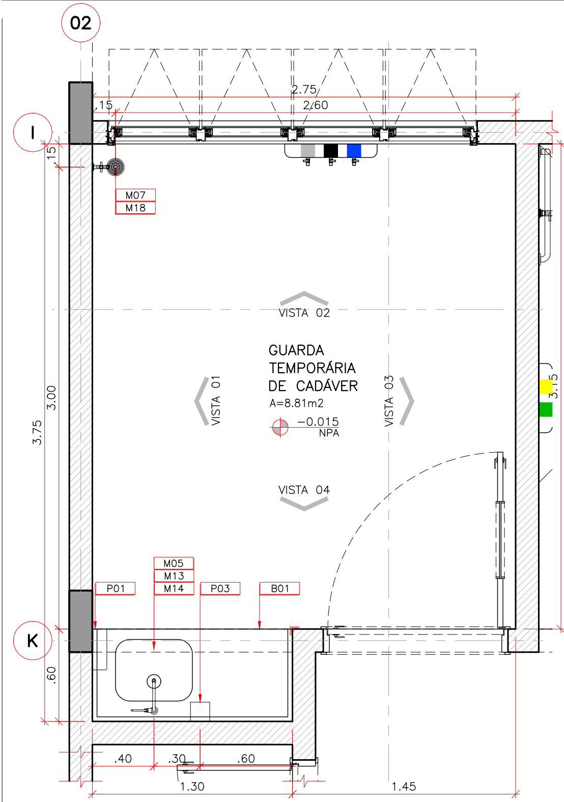
01 UNIDADE DE PRONTO ATENDIMENTO – PORTE 1 GUARDA TEMPORÁRIA DE CADAVER ESCALA: 1:25
