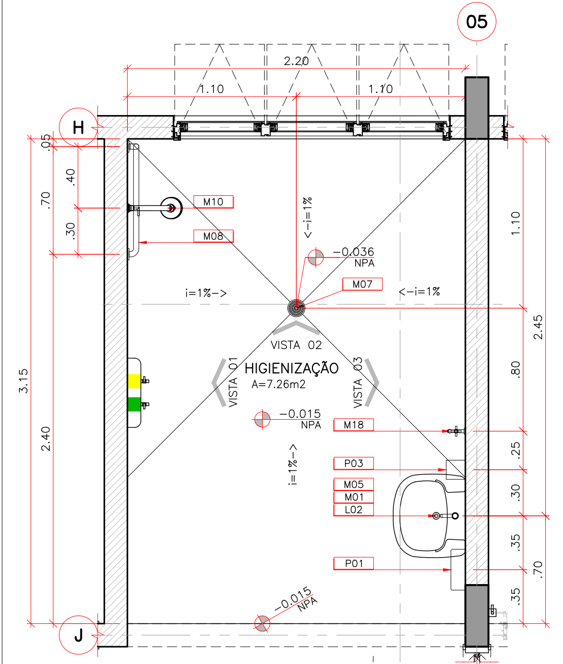
03 UNIDADE DE PRONTO ATENDIMENTO – PORTE 1 HIGIENIZAÇÃO ESCALA: 1:25
