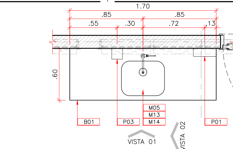
04 UNIDADE DE PRONTO ATENDIMENTO – PORTE 1 BANCADA 02 ESCALA: 1:25
