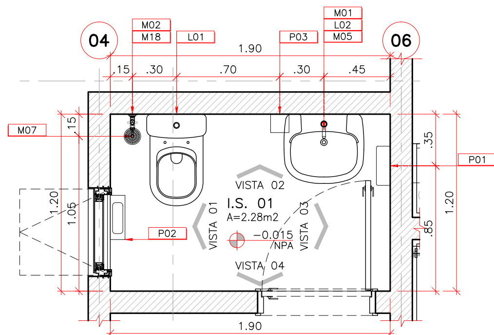
02 UNIDADE DE PRONTO ATENDIMENTO – PORTE 1 I.S. 01 ESCALA: 1:25
