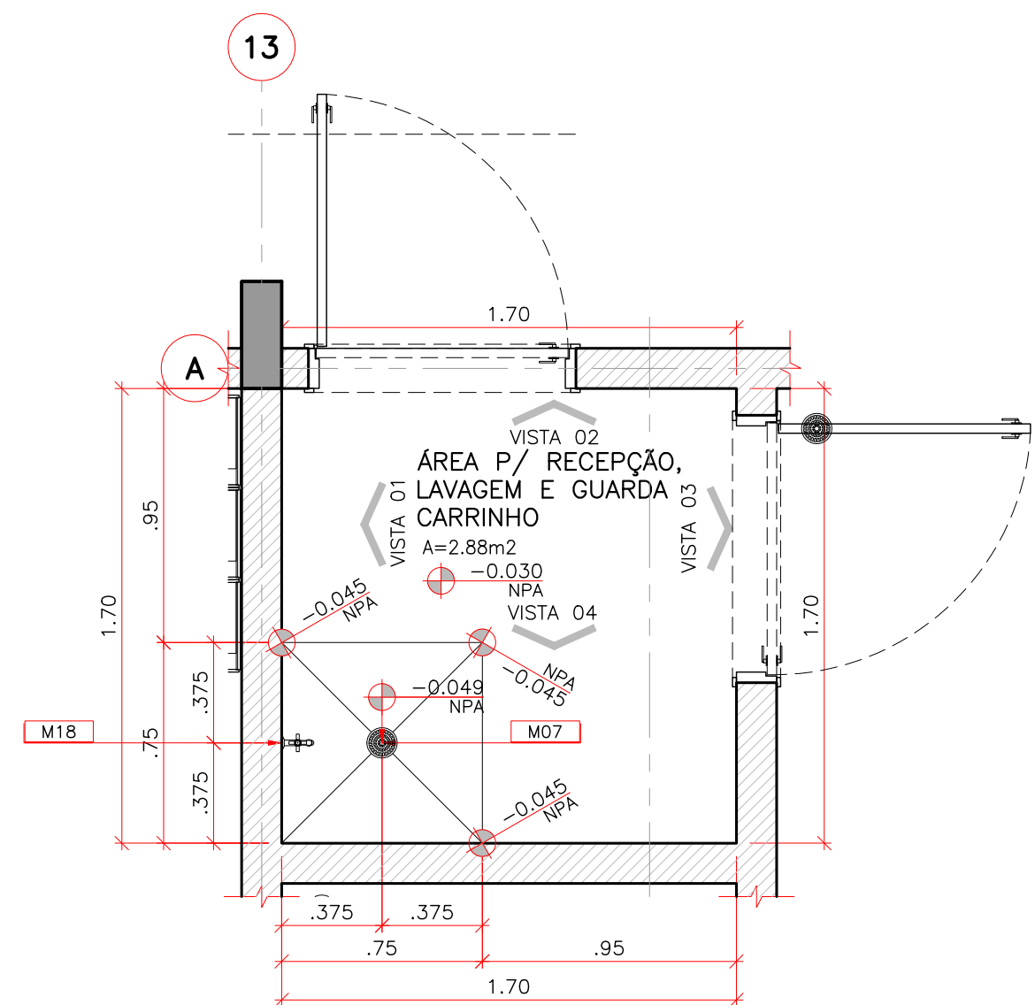
05 UNIDADE DE PRONTO ATENDIMENTO – PORTE 1 ÁREA P/ RECEPÇÃO, LAVAGEM E GUARDA CARRINHO ESCALA: 1:25
