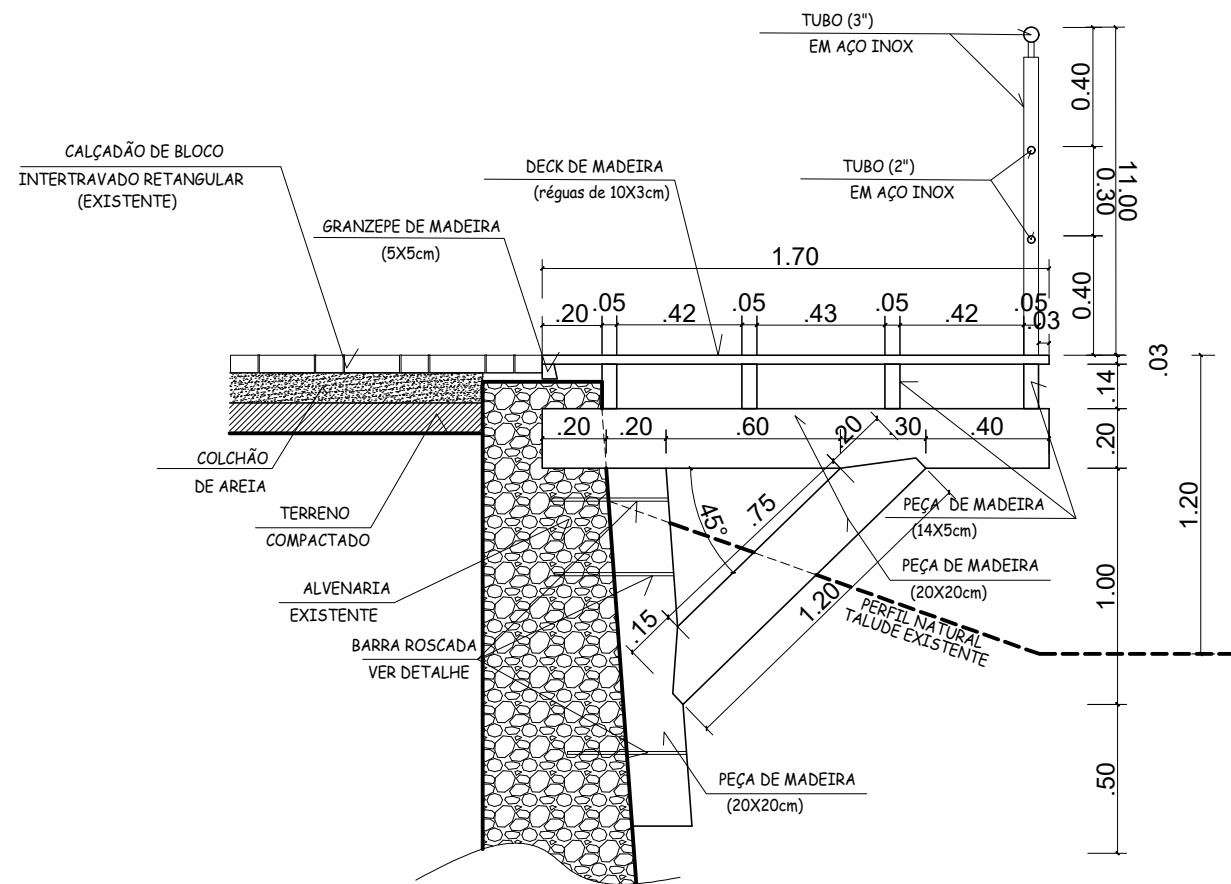
SEÇÃO - ETAPA A e B ESC. 1/125
