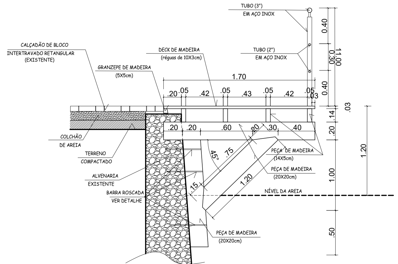
SEÇÃO - ETAPA C, E e F ESC. 1/125
