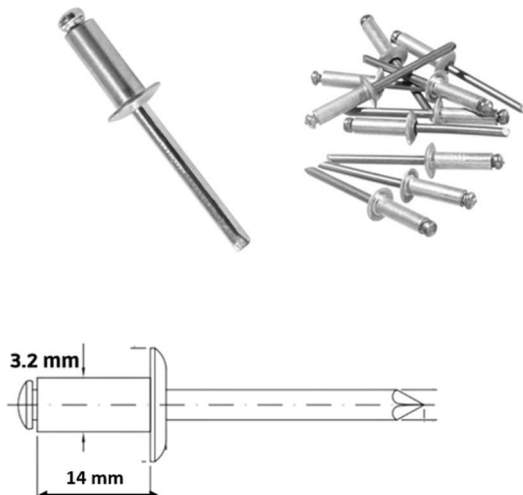
Foto Ilustrativa Item 02: rebite “pop” de alumínio nº 314
