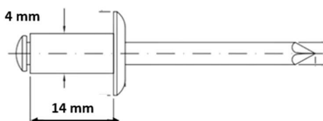
Foto Ilustrativa Item 04: rebite “pop” de alumínio nº 414
