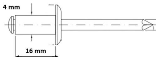
Foto Ilustrativa Item 05: rebite “pop” de alumínio nº 416
