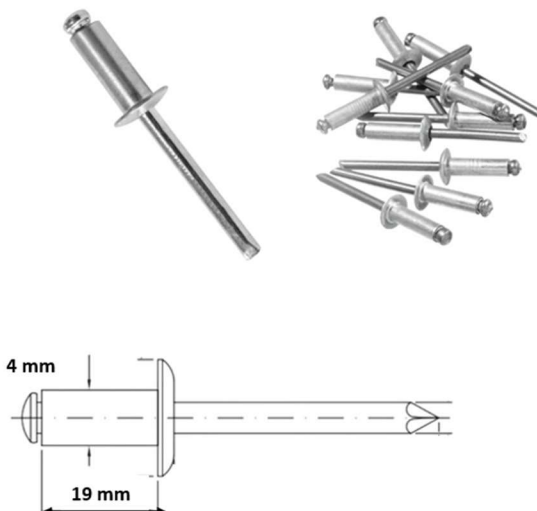
Foto Ilustrativa Item 06: rebite “pop” de alumínio nº 419
