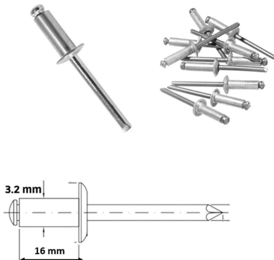
Foto Ilustrativa Item 03: rebite “pop” de alumínio nº 316
