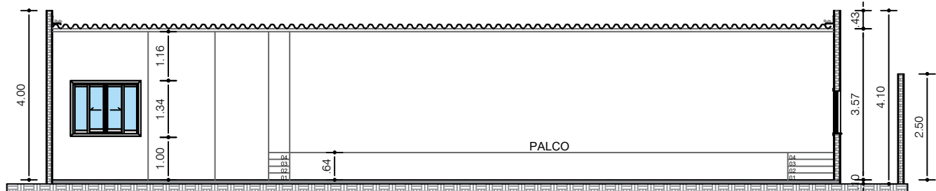
CORTE A/A
