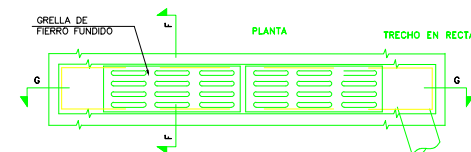
CORTE GG
