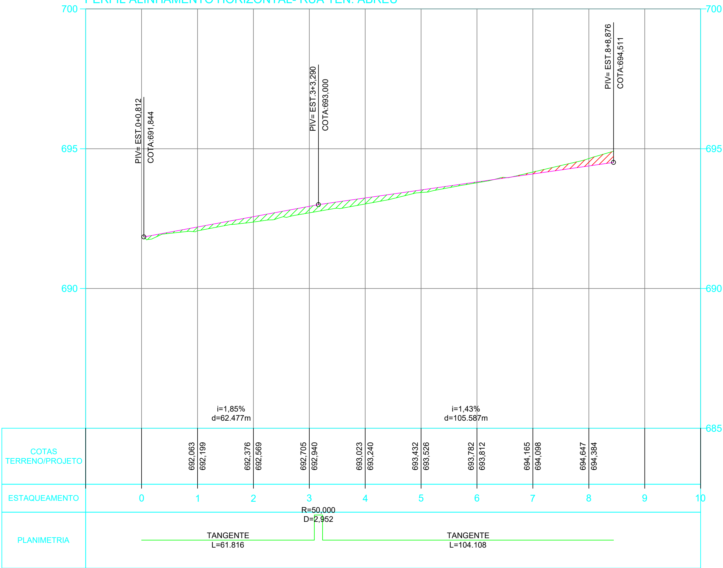
PERFIL ALINHAMENTO HORIZONTAL- RUA TEN. ABREU
