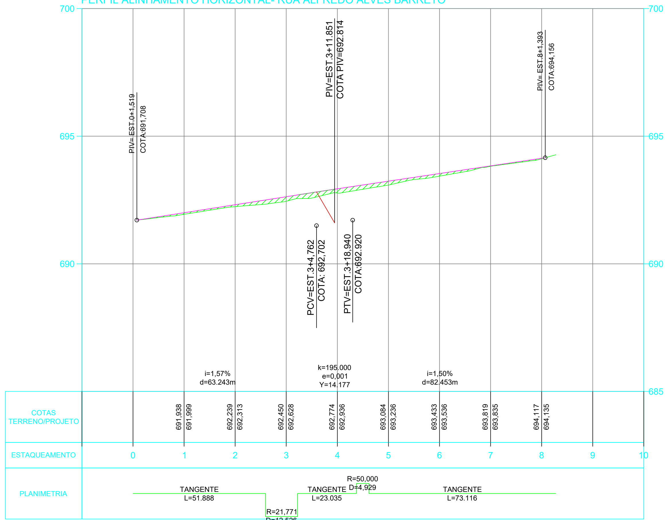
PERFIL ALINHAMENTO HORIZONTAL- RUA ALFREDO ALVES BARRETO
