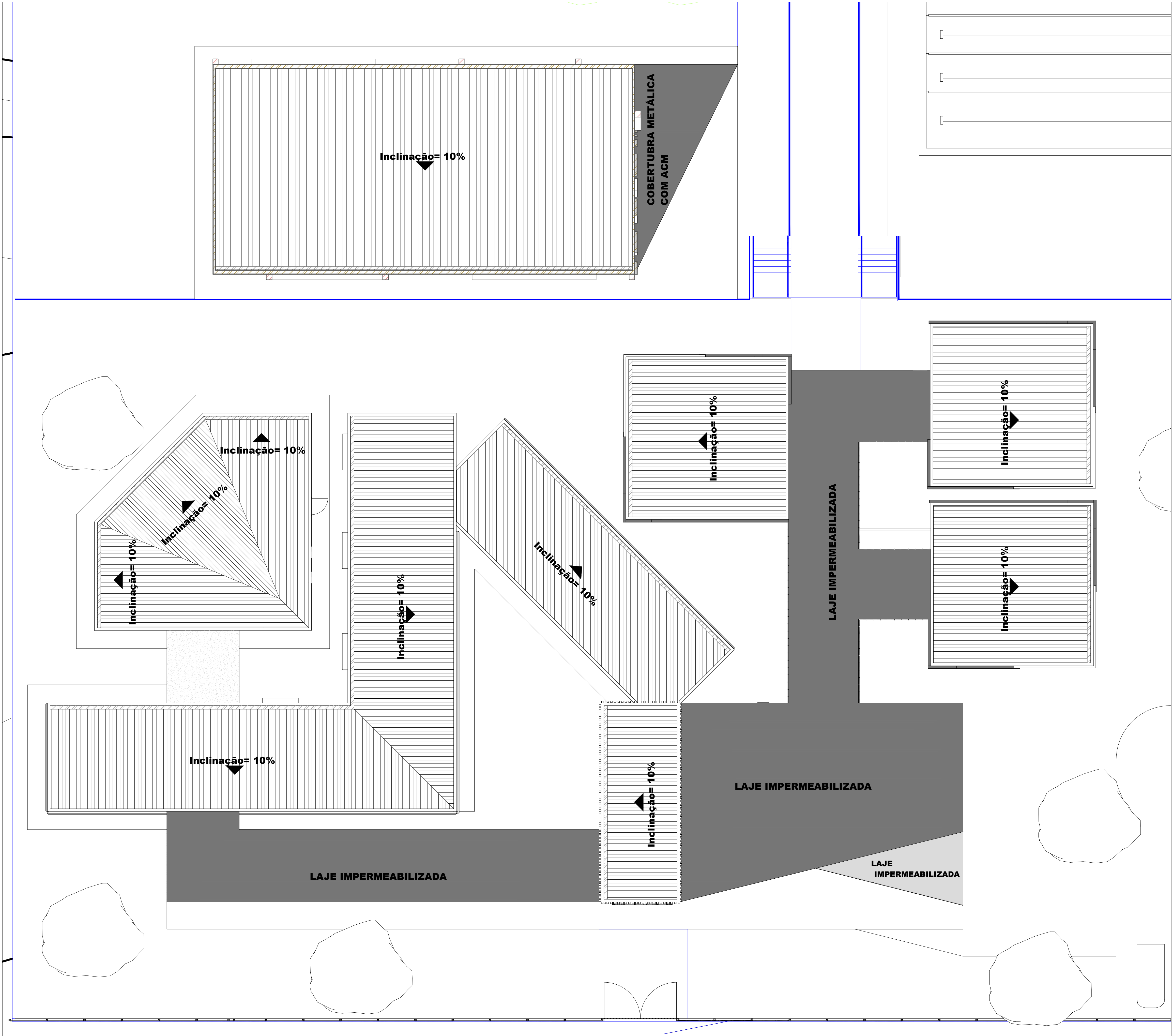
1 PLANTA BAIXA 1 : 75
