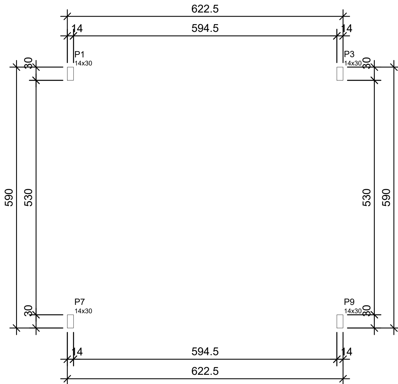
Forma do pavimento Laje (Nível 375) escala 1:50
