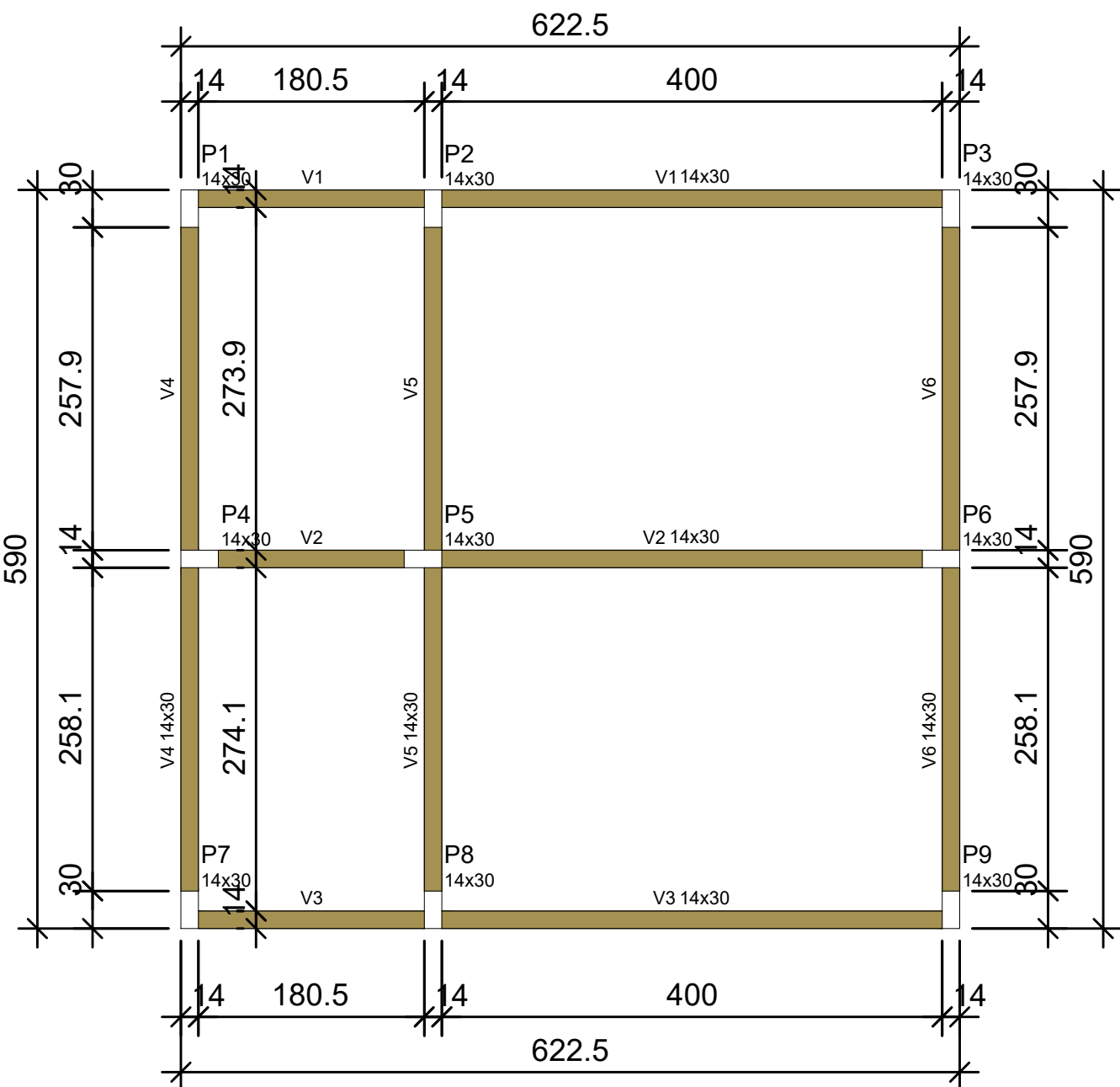
Forma do pavimento Térreo (Nível 0) escala 1:50
