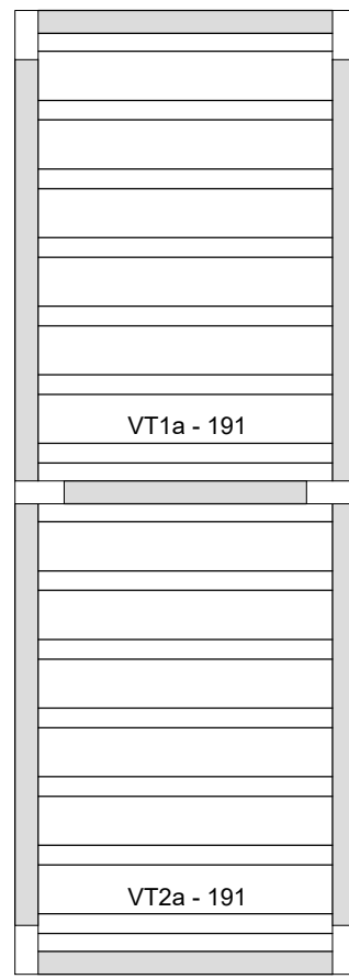
Planta de vigotas pré-moldadas escala 1:50
