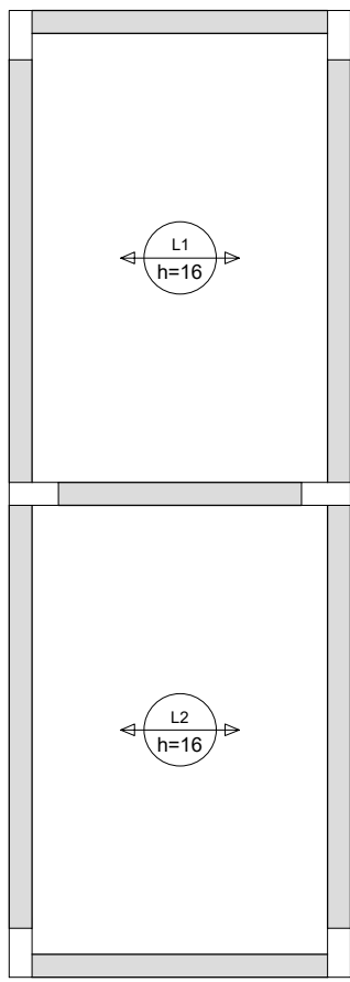
Armação positiva das lajes do pavimento Cobertura (Eixo X) escala 1:50
