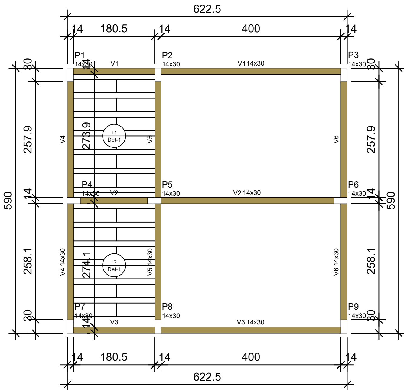
Forma do pavimento Cobertura (Nível 300) escala 1:50
