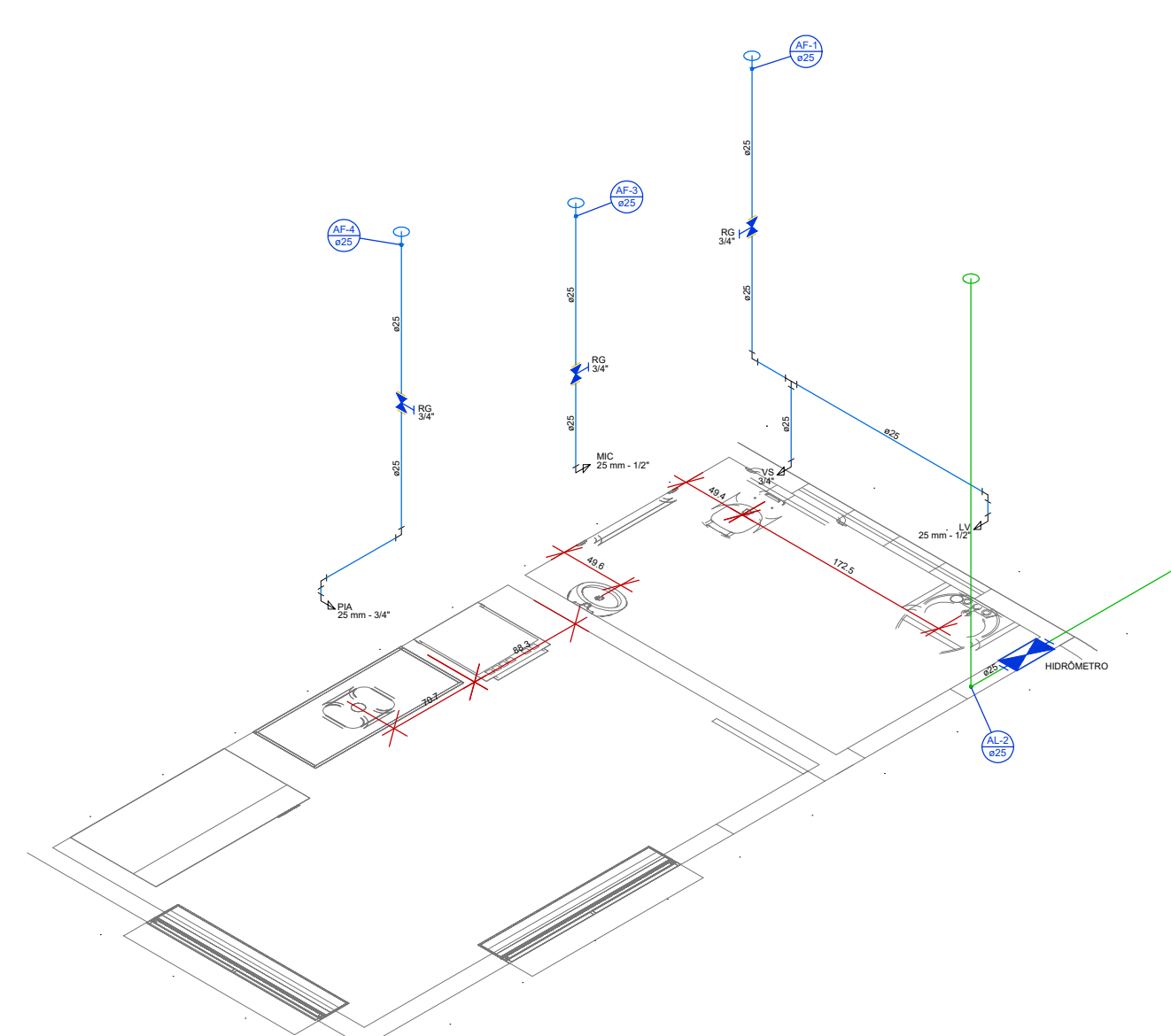
Detalhe H2 Escala 1:25
