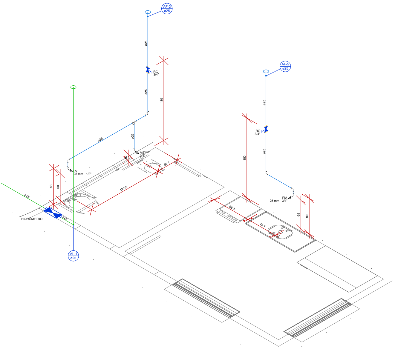
Detalhe H1 Escala 1:25
