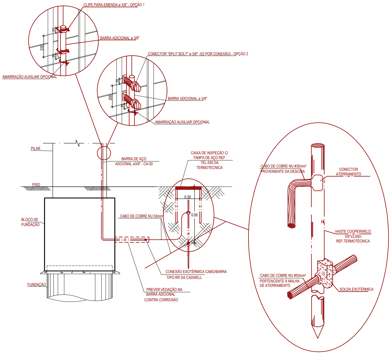
DETALHE ATERRAMENTO NOS PILARES INDICADOS EM PLANTA, COM CAIXA DE INSPEÇÃO SEM ESCALA
