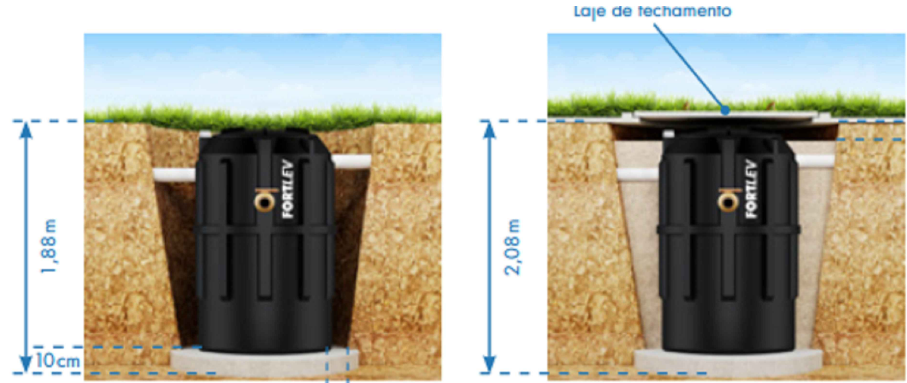
Figura 3 – Instalação sem laje de fechamento.
