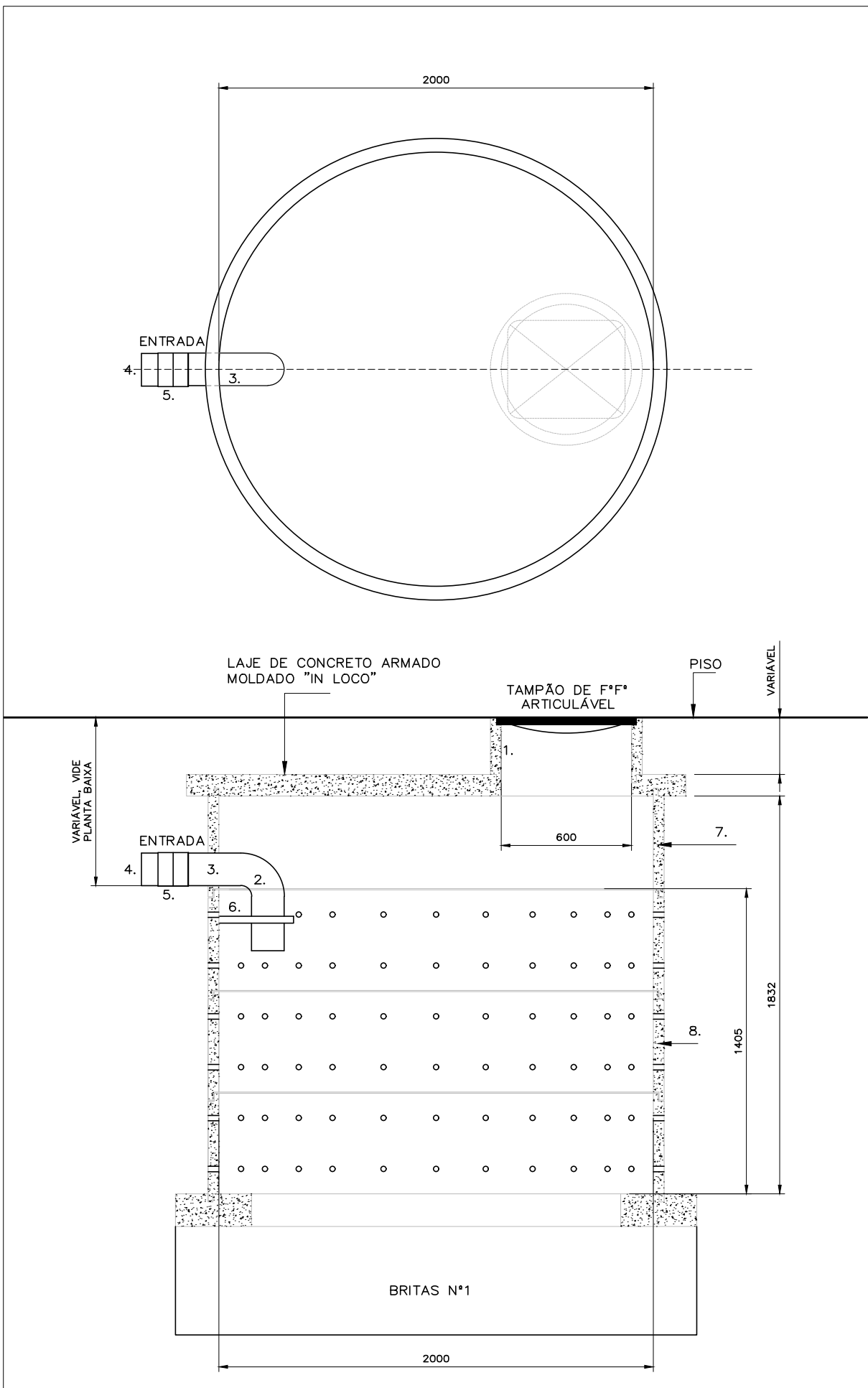
SUMIDOURO Escala: 1/25 Cotas em mm.
