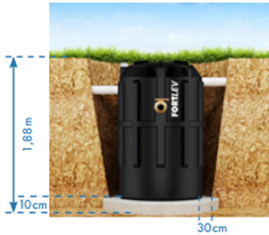
Figura 3 - Instalação sem laje de fechamento.
