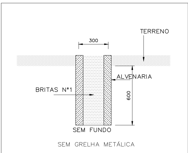
VALA DE INFILTRAÇÃO Cotas em mm. Escala: 1/20
