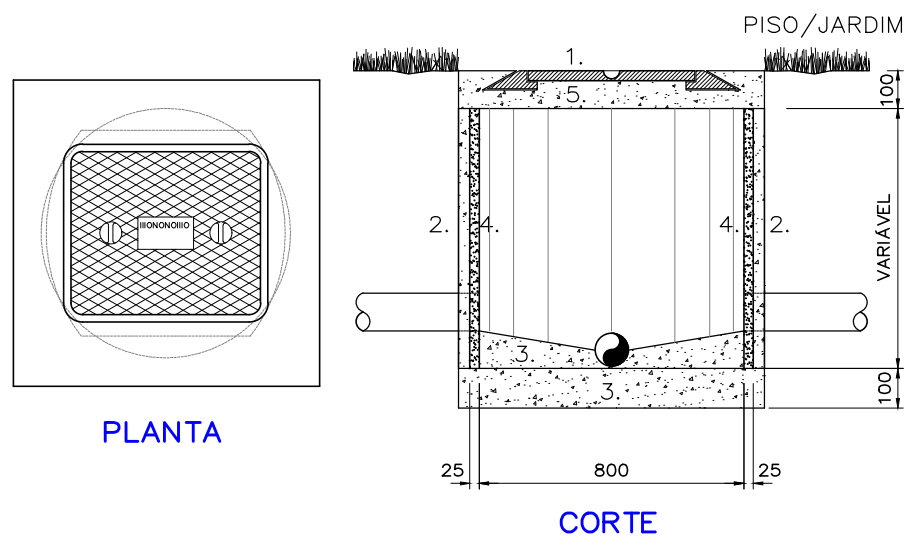
CAIXA DE INSPEÇÃO Ø700 ESC. 1/20
