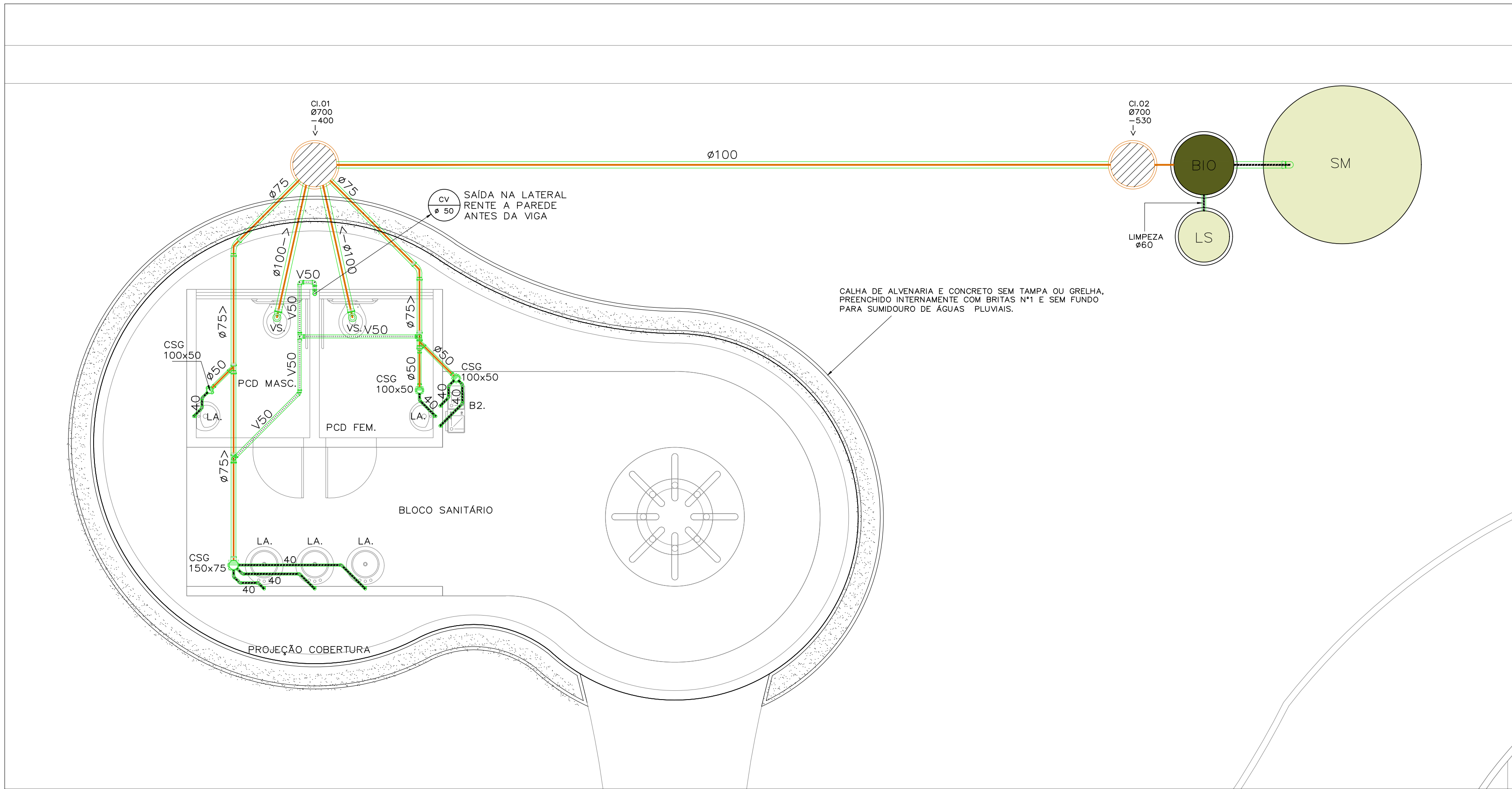
PLANTA BAIXA MÓDULO SANITÁRIO Cotas em mm. Escala: 1/50
