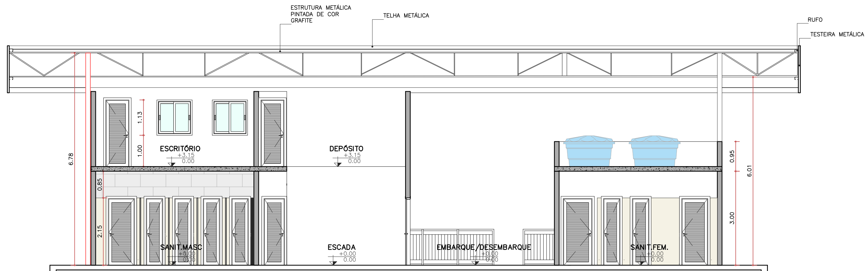
CORTE A ESC. 1:75
