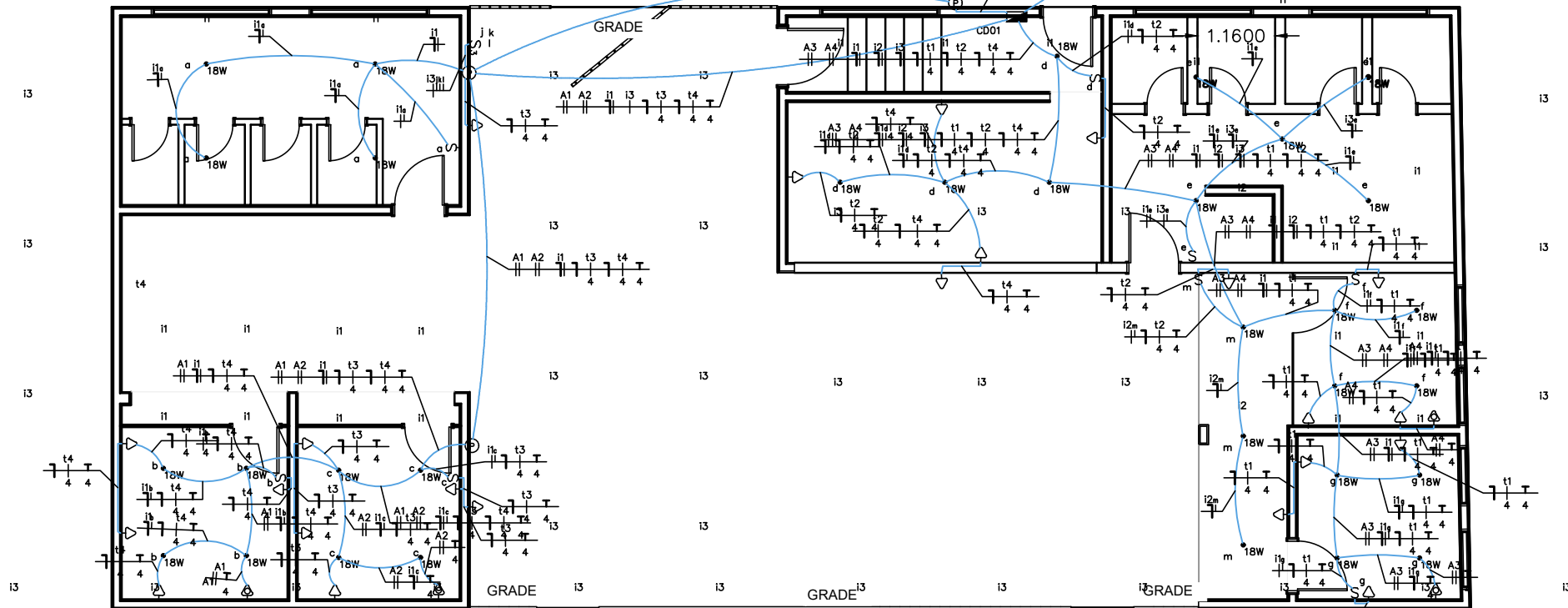
PLANTA TERREO ESC:1/50
