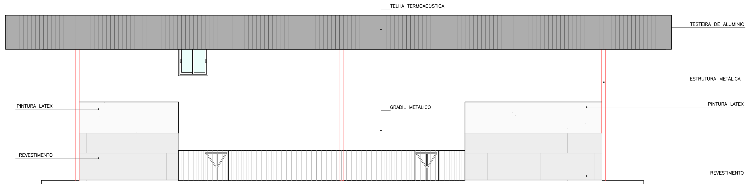
VISTA A ESC. 1:75
