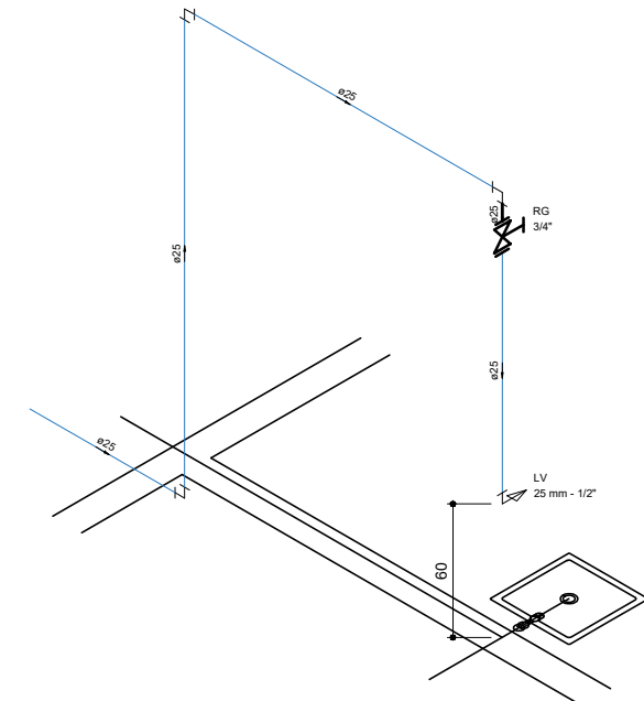
Detalhe H3 escala 1:25
