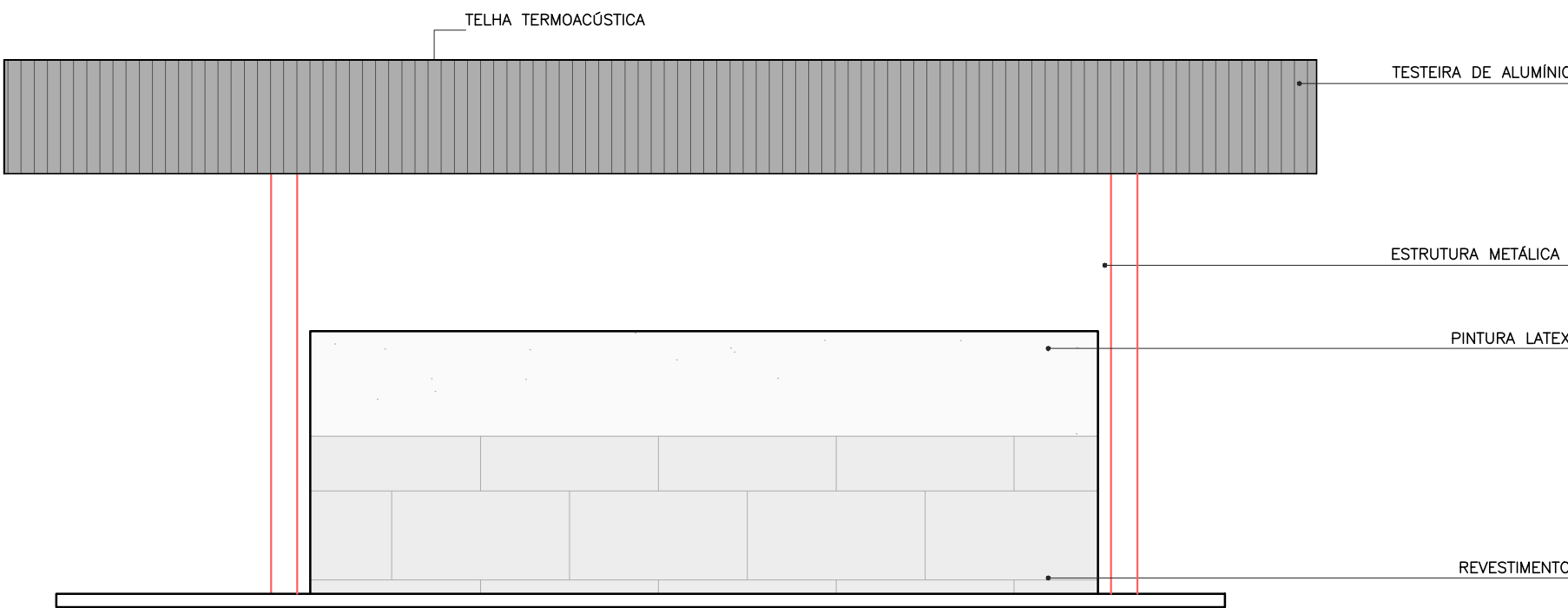
VISTA B ESC. 1:75
