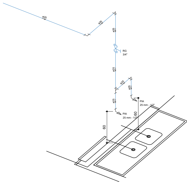
Detalhe H2 escala 1:25
