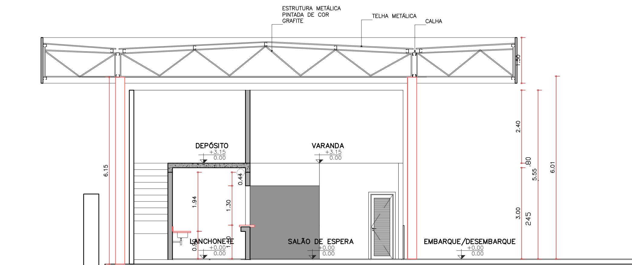
CORTE B ESC. 1:75
