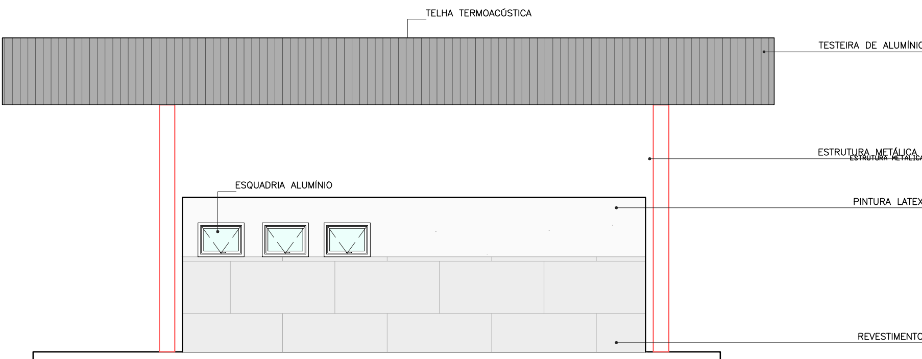
VISTA D ESC. 1:75
