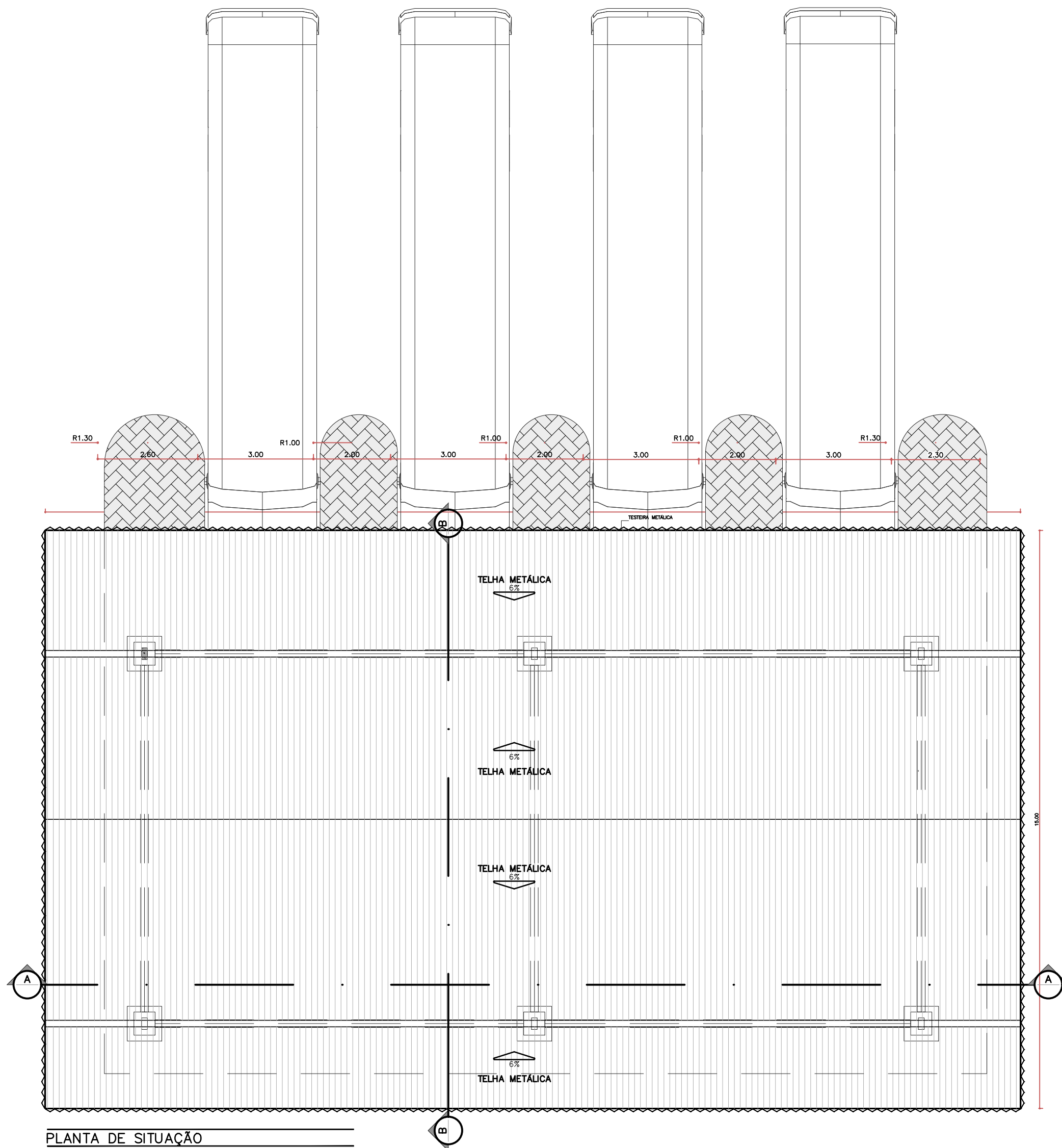
PLANTA DE SITUAÇÃO ESC. 1:50
