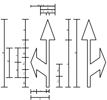
SETA INDICATIVA DE MUDANÇA OBRIGATÓRIA DE FAIXA
