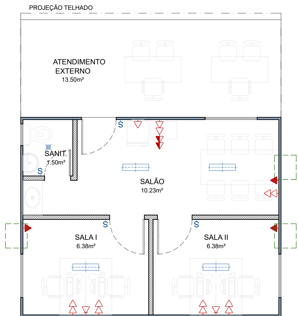
PLANTA DE PONTOS ELÉTRICOS, ILUMINAÇÃO E AR CONDICIONADO ESC.: 1/50
