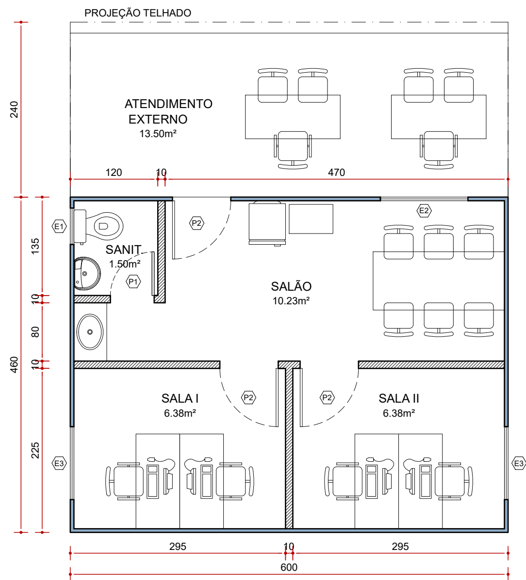
PLANTA DE LAYOUT ESC.: 1/50
