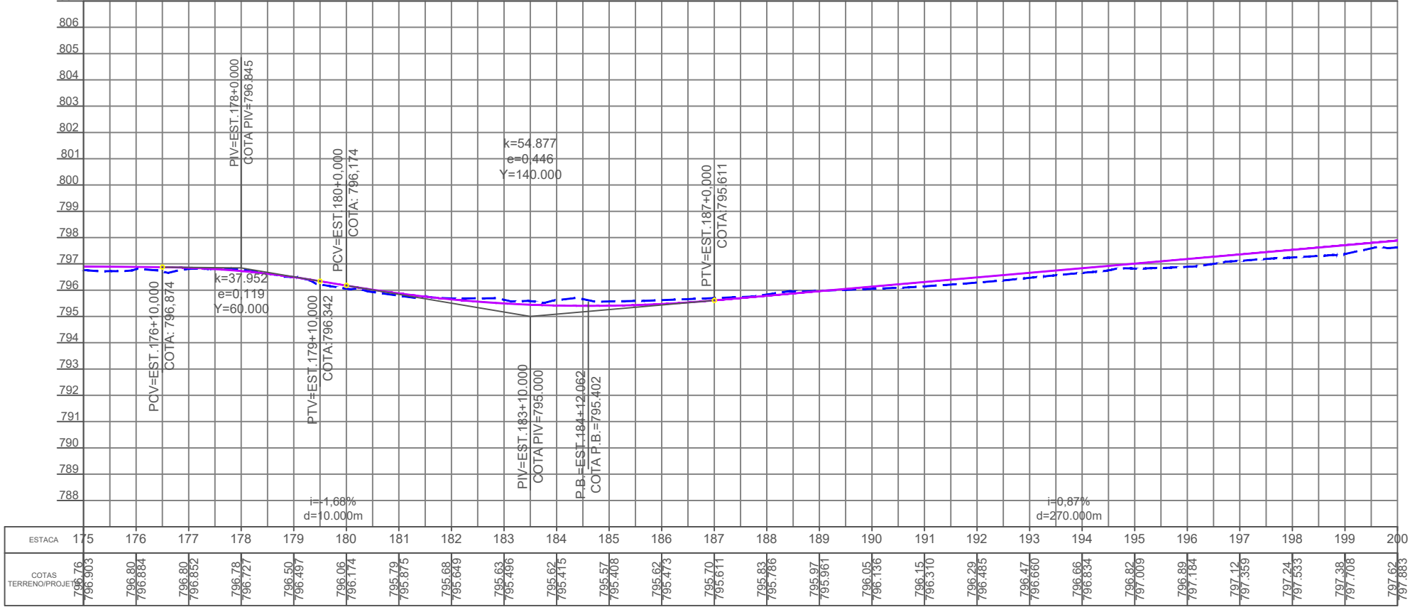
807 PERFIL EIXO BA -434
