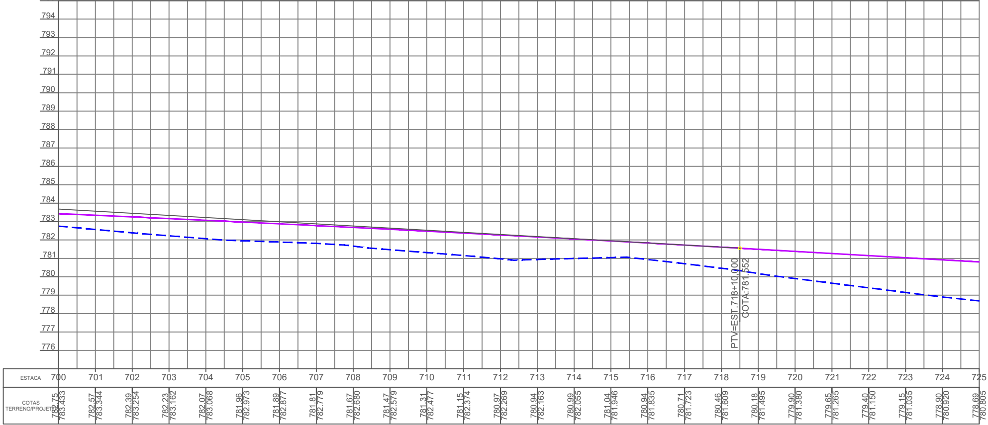
795 PERFIL EIXO BA -434
