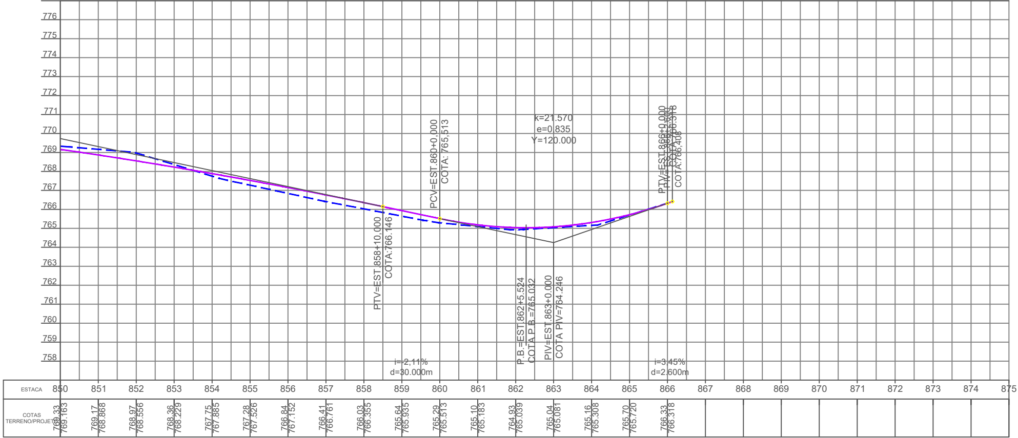
777 PERFIL EIXO BA -434
