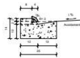
Seção transversal Escala 1:10
