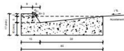
Seção transversal Escala 1:10
