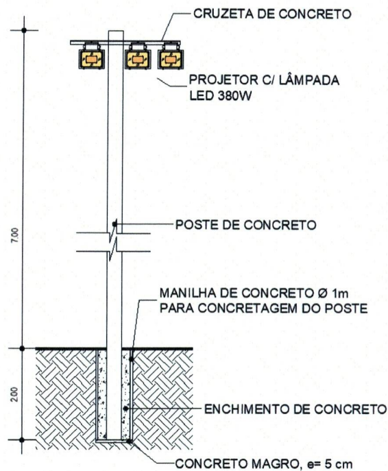
Figura 06 – Vista frontal do sistema de iluminação em LED
