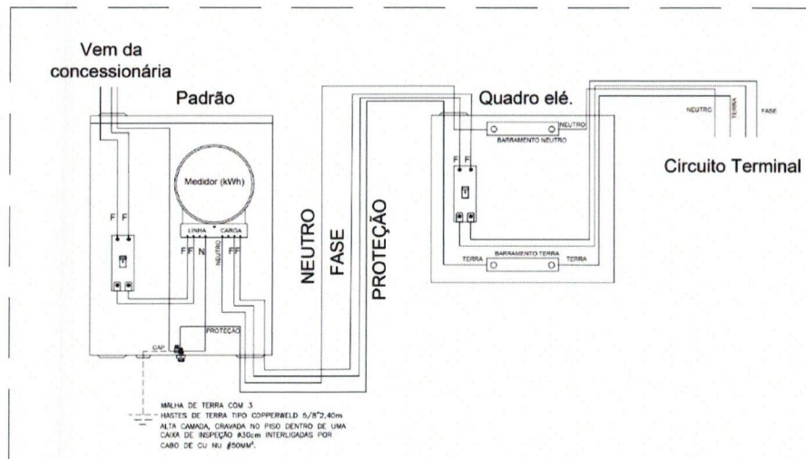
Figura 05 – Esquema TN-S_Detalhe da instalação do medidor de energia e do Quadro de distribuição Sistema Bifásico
