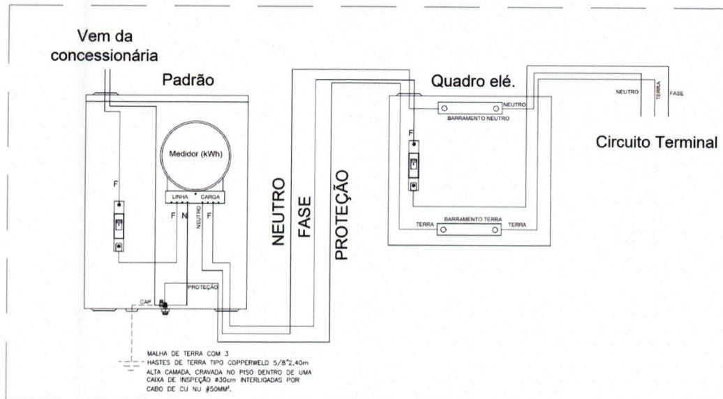
Figura 04 – Esquema TN-S_Detalhe da instalação do medidor de energia e do Quadro de distribuição Sistema Monofásico
