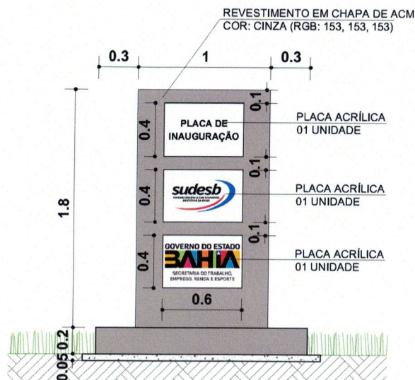
Figura 07 – Totem padrão SUDESB Fonte: Elaborado pelo autor, SUDESB (2023).
