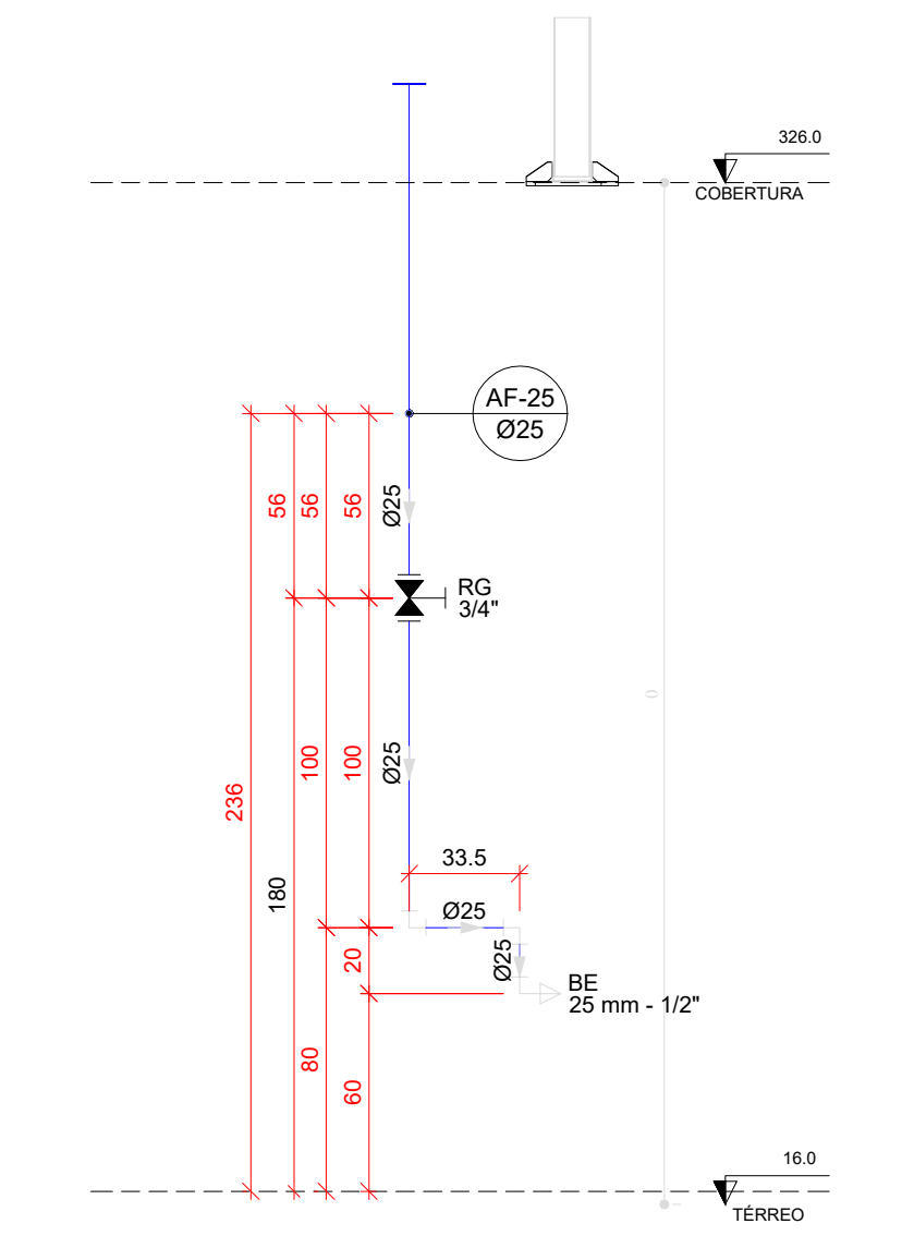
H34 DETALHE H34 ESCALA 1/25
