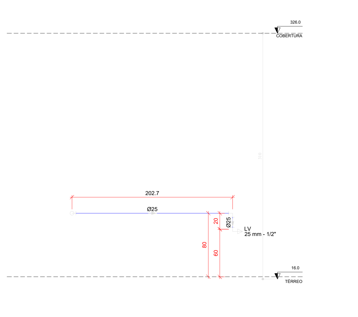
H29 DETALHE H29 ESCALA 1/25
