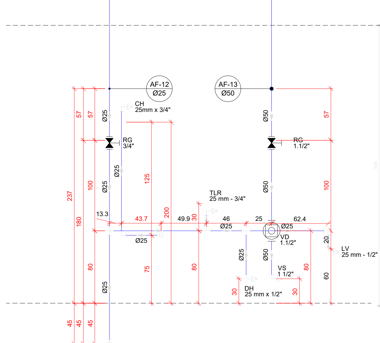
H24 DETALHE H24 ESCALA 1/25
